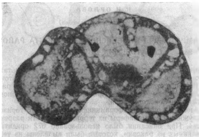
Фиг. 2. Endothyranopsis ex. gr. crassus (Brady). Скошенное поперечное сечение. В стенке раковины хорошо видны крупные зерна кальцита и кварца. Оригинал № 45, фото; \times 115 .
