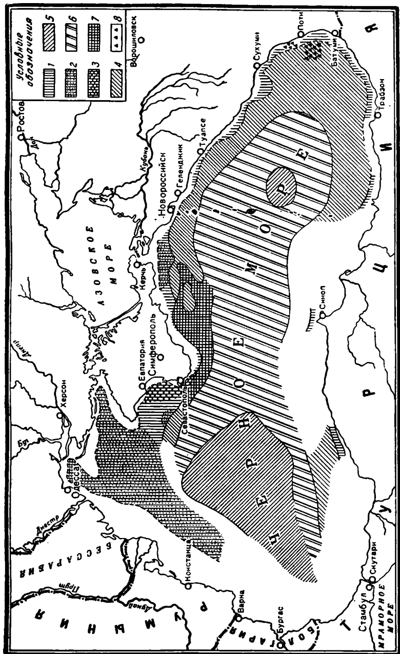
Фиг. 14. Схема распределения осадков Древнечерноморского бассейна.
