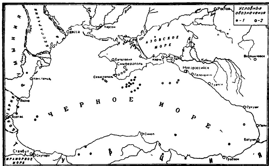
Фиг. 6. Эпицентры, отмеченные крымскими станциями с 1928 по 1932 г.; по Полумбу [118].
