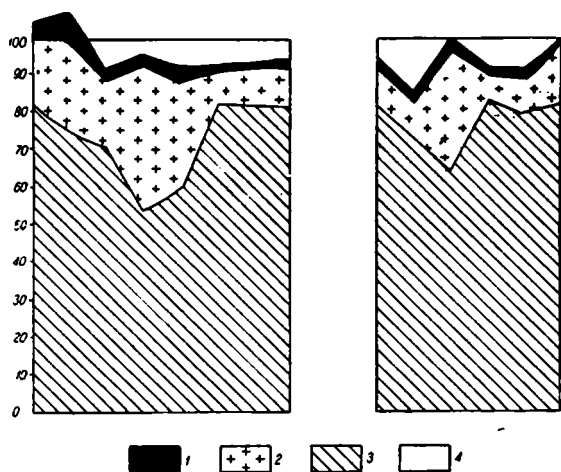
Фиг. 8. Основные компоненты мидиевого (слева) и фазеолинового (справа) илов. 1 — органическое вещество; 2 — карбонаты; 3 — обломочный материал; 4 — прочее (вода, минеральные новообразования и т. п.). Цифры слева — проценты.
