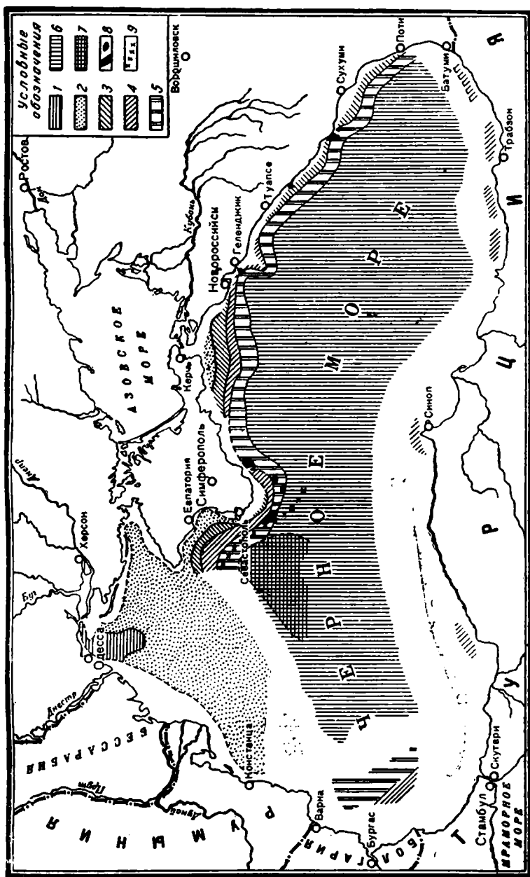
Фиг. 24. Новоевксинский бассейн
