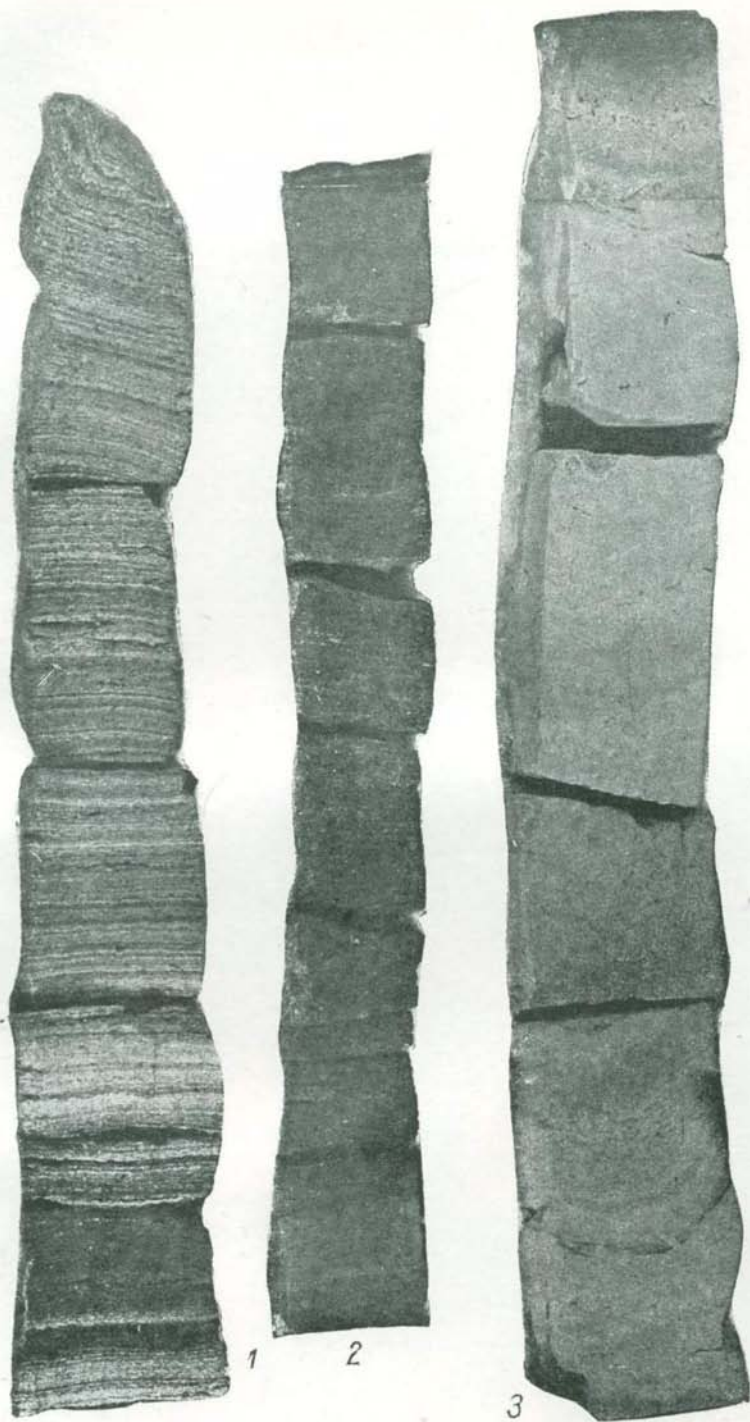
Колонка черноморского ила из глубоководной области, разрезанная на составные части (уменьшение \frac{4}{5} ).
