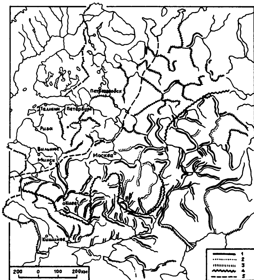
Рис. 5. Схема крутизны склонов долин европейской части СССР.
