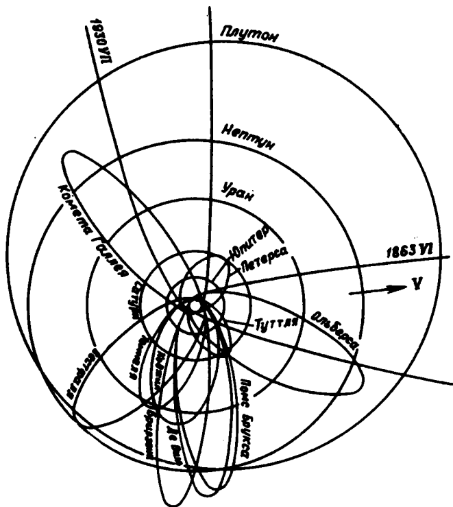
Рис. 11. Орбиты некоторых периодических комет семейства Сатурна, Урана, Нептуна.
