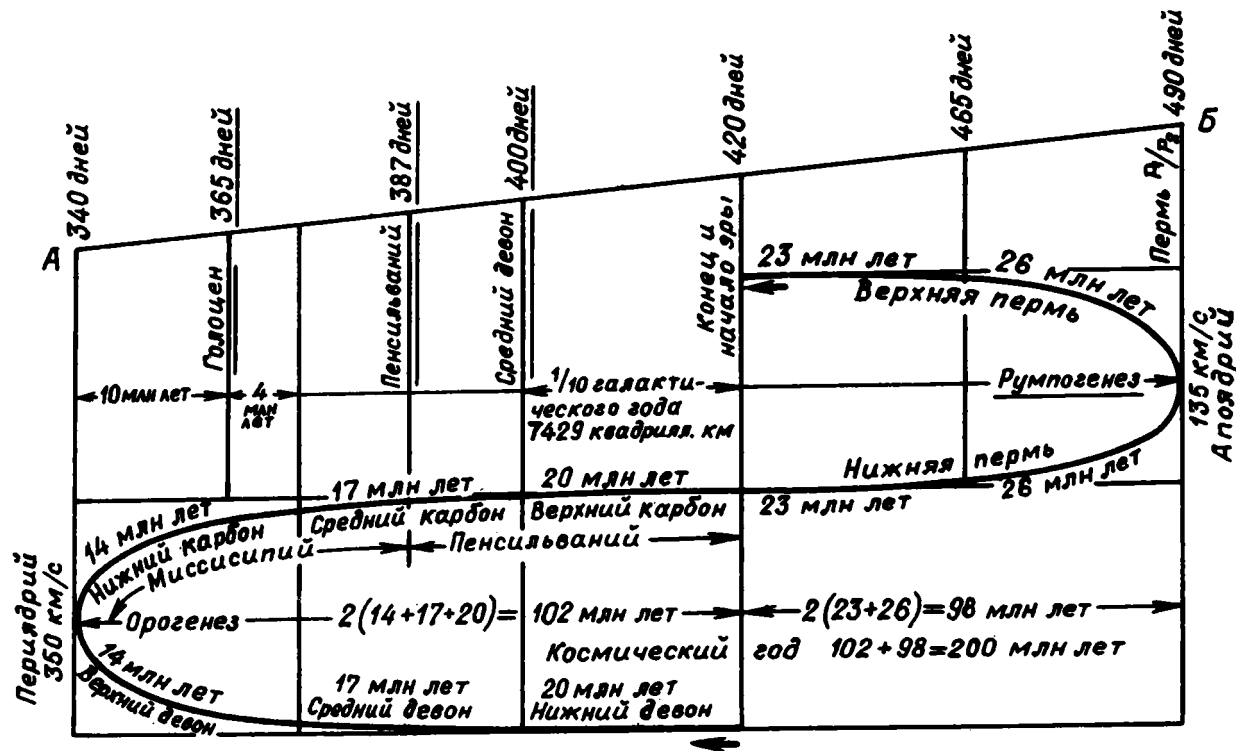
Рис. 29. Определение продолжительности земного года (скорость ротации Земли).
