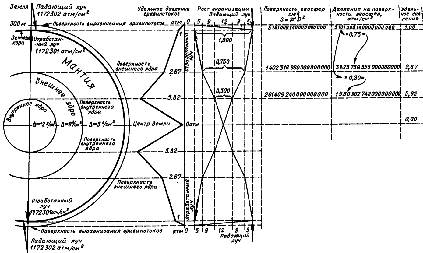
Рис. 18. Расчет давления гравитационных потоков внутри Земли.
