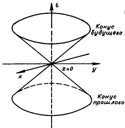
Рис. 20. Пространственно-временной мир по А. Эйнштейну.
