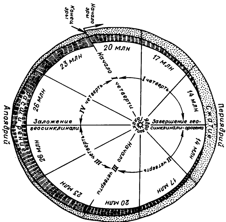
Рис. 25. Фоновое развитие тектоники на Земле по геокалендарю.
