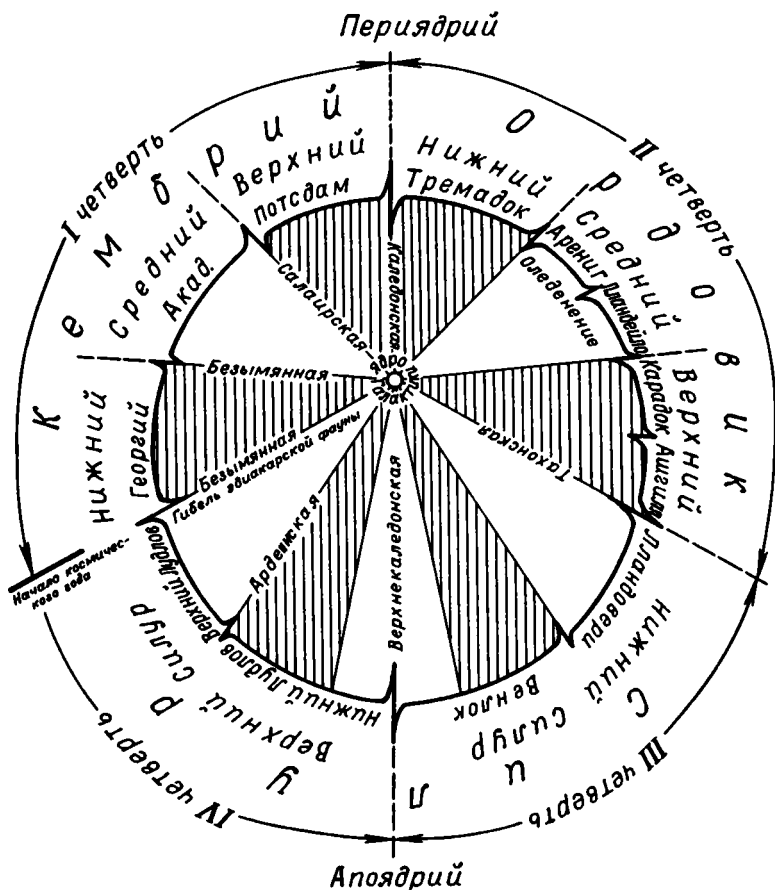
Рис. 31. Геокаленды нижнего палеозоя.
