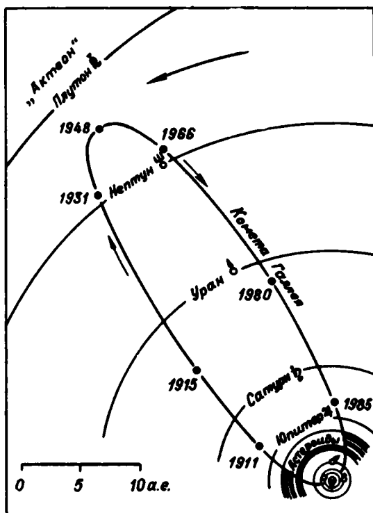
Рис. 16. План Солнечной системы (комета Галлея, возможно, результат взрыва планеты Актеон).
