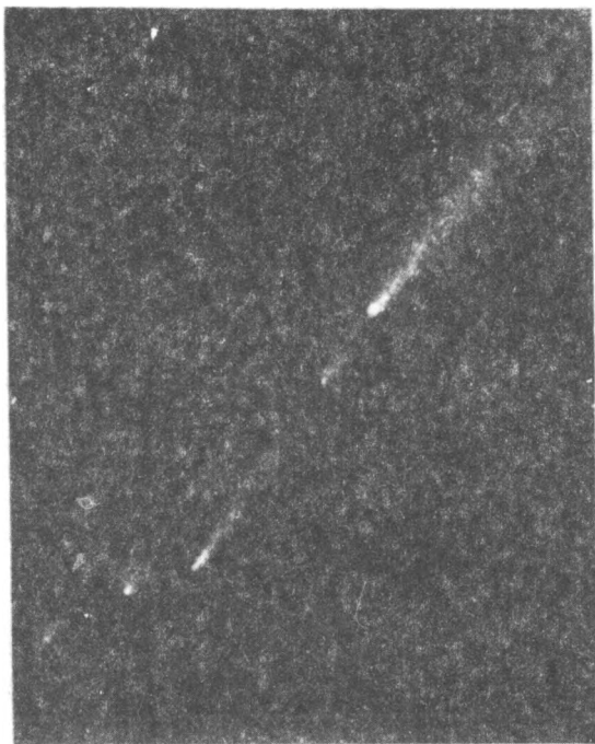
Рис. 23. Распад кометы Брукса (1889 V).
