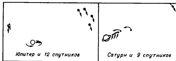
Рис. 6. Солнечная система — гигантское завихрение гравитационных потоков.
