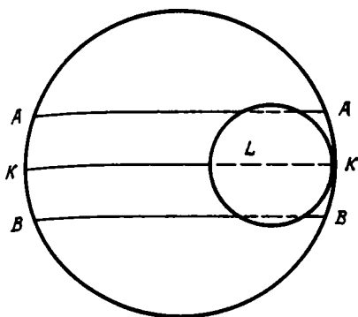
Рис. 19. Опыт Гюйгенса. Цилиндрический сосуд с водой и шарик с удельным весом, равным удельному весу воды, движущиеся между тремя струнами AA, KK и BB.
