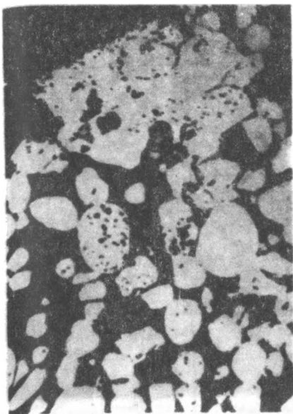
Рис. 34. Микрофотография докембрийского пирито-кварцевого песка из системы Витватерсранд, Южная Африка (Ув. \times 45 ).
