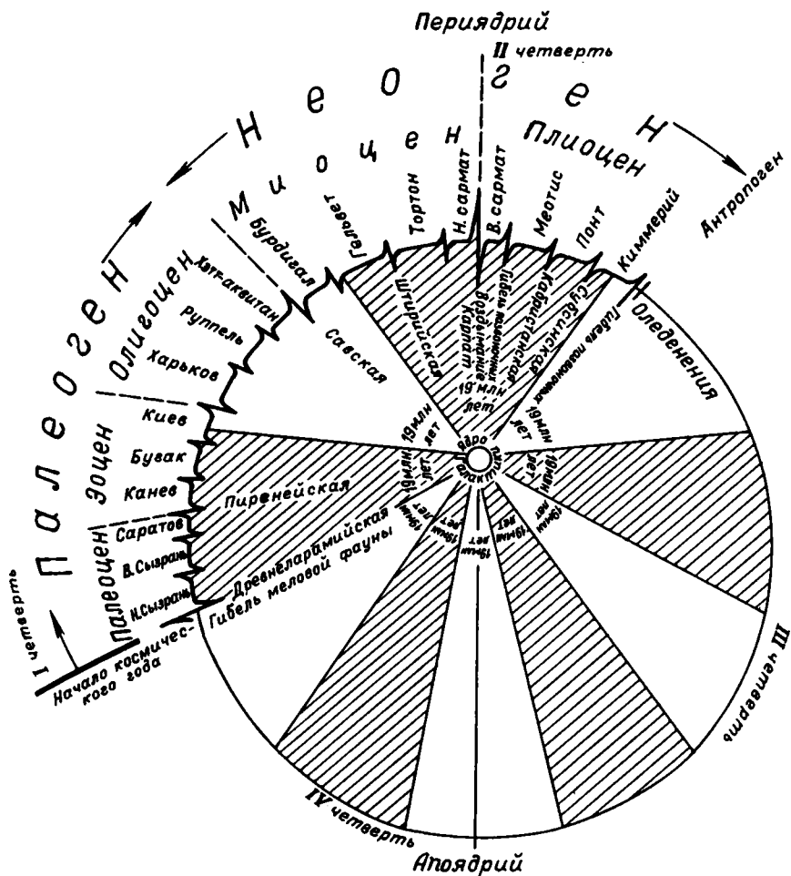
Рис. 26. Геокаленды кайнозоя.
