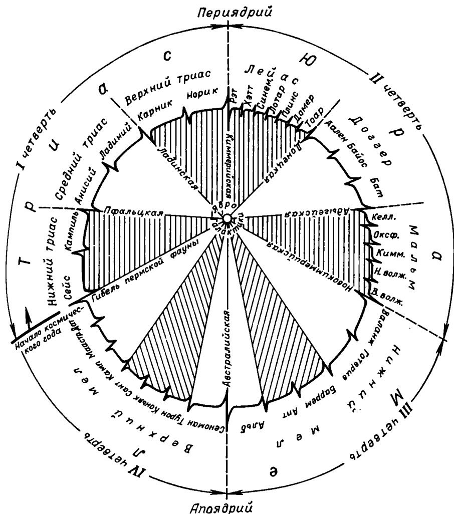
Рис. 27. Геокаленды мезозоя.
