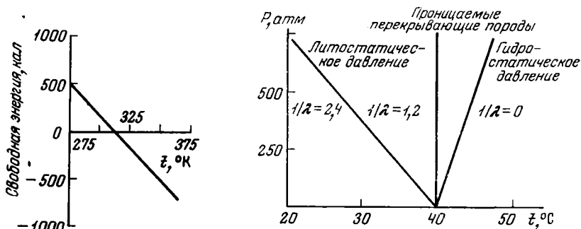
Рис. 8. Зависимость свободной энтальпии реакции обезвоживания гипса в воде от температуры (по Р. Керну и А. Вайсброду, 1966)
