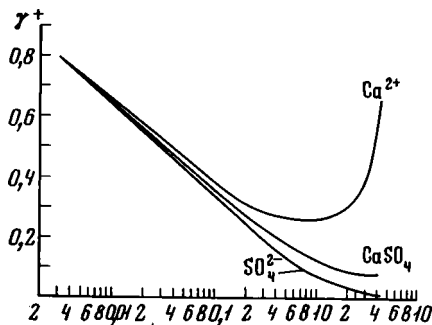
Рис. 13. Кривые зависимости коэффициентов активности ионов \text{Ca}^{2+} и \text{SO}_4^{2-} и среднего коэффициента активности \text{CaSO}_4 от ионной силы раствора
