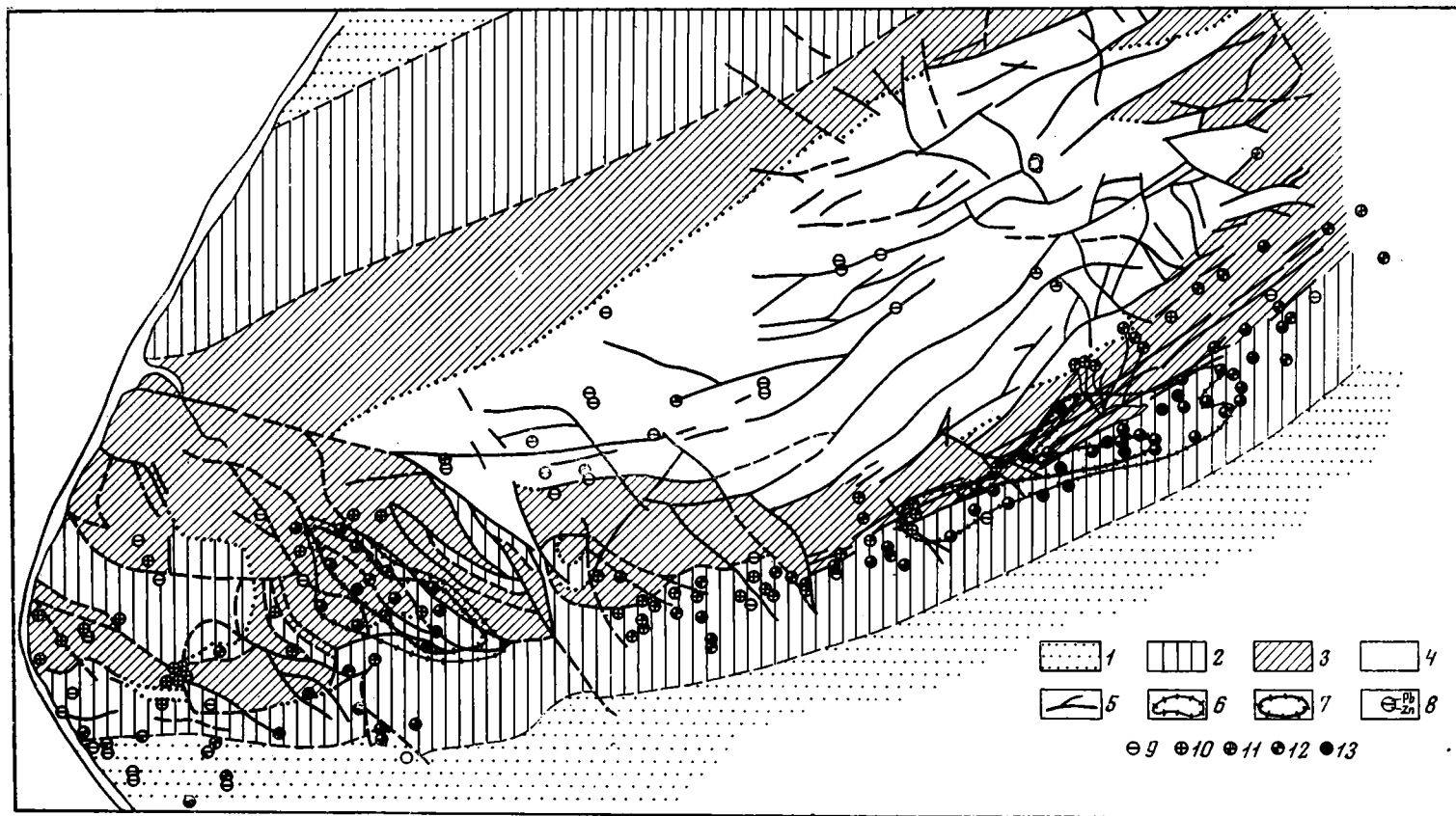
Рис. 48. Схема гидрогеохимических и гидротермических аномалий п-ва Челекен (геологическая основа по А. С. Архипченко)
