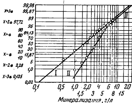
Рис. 40. Вероятностный график распределения минерализации вод сенона и верхнего тулона в областях питания (I) и разгрузки (II) подземных вод
