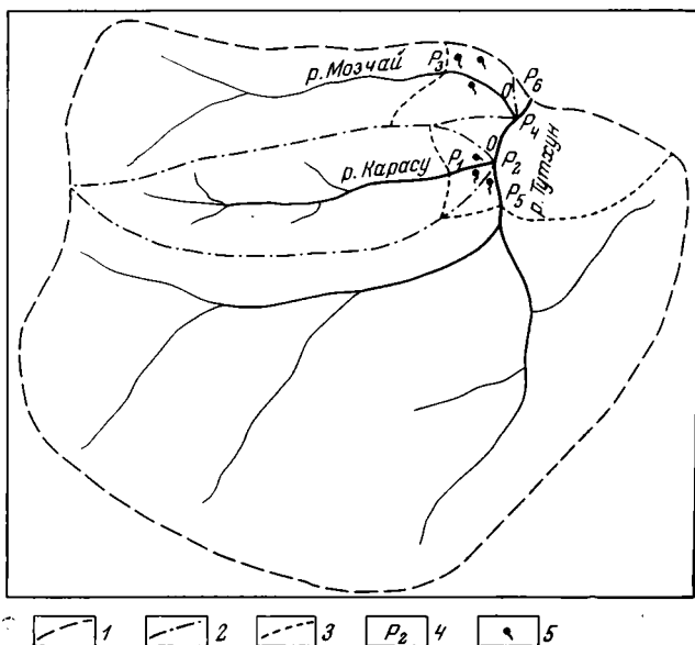
Рис. 36. Схема бассейна р. Тутхун (в границах изученной его части)
