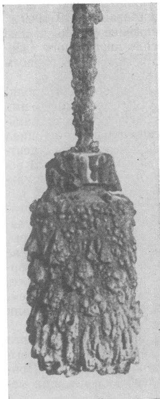
Рис. 58. Натечные образования геля сульфида железа на затравках, возраст 6 месяцев (натуральная величина)
