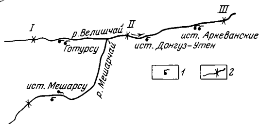
Рис. 38. Схема расположения термоминеральных источников бассейна р. Велишчай
