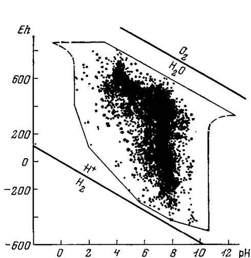
Рис. 21. Распределение значений Eh и pH в природных водных средах (по Л. Г. Басс-Бекингу, Л. Р. Каплану и Д. Муру, 1963)
