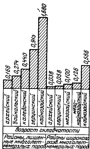
Рис. 32. Средневзвешенные по стоку модули подземного химического стока для разновозрастных структур
