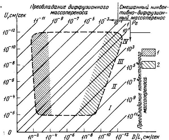
Рис. 28. Схема распределения полей преобладания конвективного и диффузионного режимов массопереноса в координатах: скорость движения подземных вод, V и коэффициент массоотдачи, D/L
