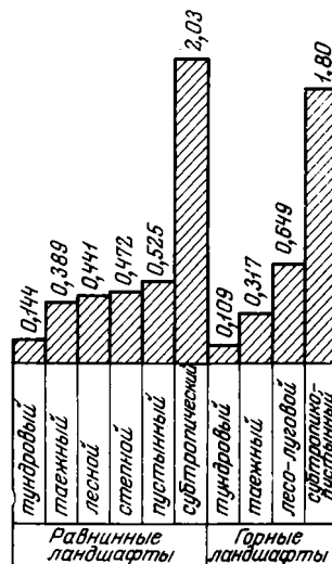
Рис. 33. Модуль подземного химического стока в различных ландшафтных зонах, г/сек \cdot км^2
