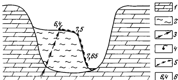
Рис. 20. Схема травертинового поля Большого Готурлинского источника в бассейне р. Тутхун 1 — коренные породы; 2 — травертины; 3 — предполагаемые пути разгрузки минеральных вод; 4 — источник; 5 — сток минеральной воды; 6 — величины рН минеральных вод
