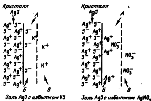
Рис. 5. Двойной электрический слой (по И. Е. Старiku, 1959)
