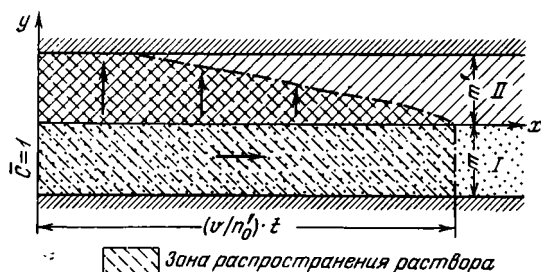
Рис. 30. Схема миграции в изолированном двухслойном пласте по В. М. Шестакову (Бочев, Гармонов, Лебедев, Шестаков, 1969)
