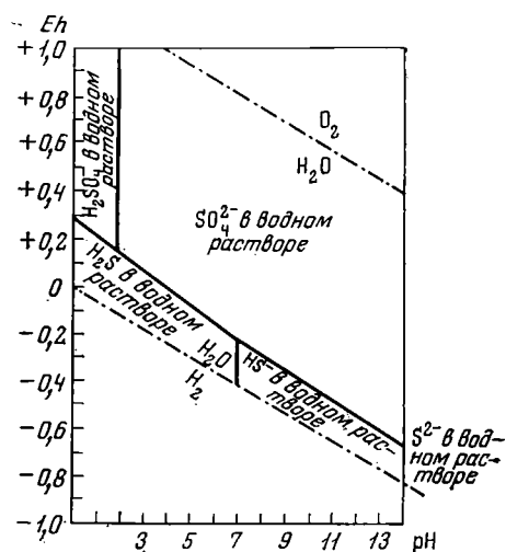
Рис. 21. Распределение значений Eh и pH в природных водных средах (по Л. Г. Басс-Бекингу, Л. Р. Каплану и Д. Муру, 1963)
