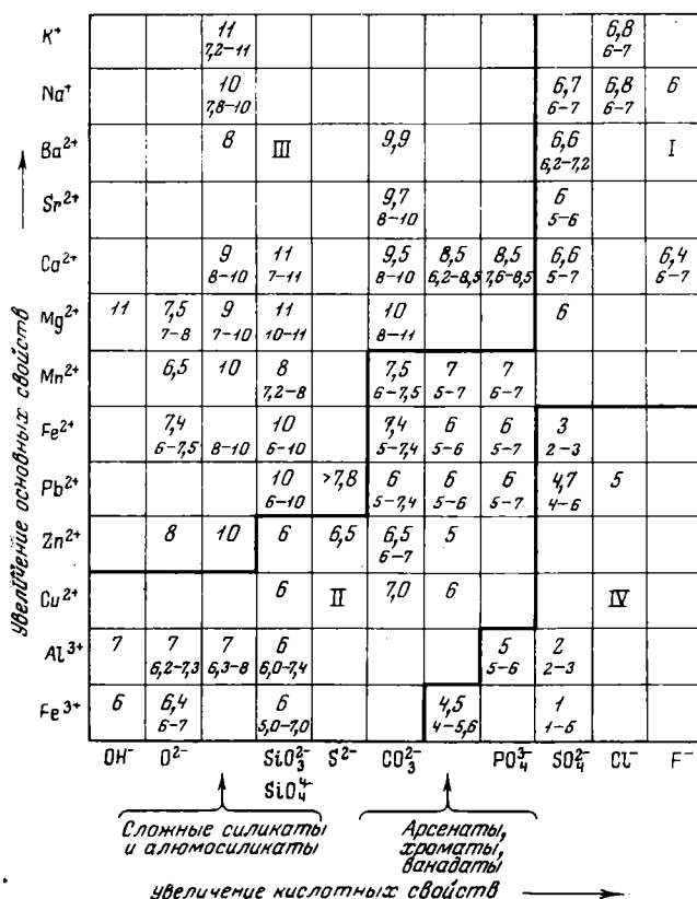
Рис. 11. Значения рН суспензий минералов (по Я. Б. Смирнову и Л. А. Матвеевой, 1963)
