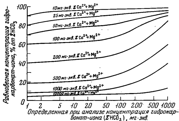
Рис. 23. Номограмма для приближенной оценки концентрации не связанных в комплексы гидрокарбонатных ионов (равновесной концентрации \text{HCO}_3^- ) в природных водах в зависимости от суммарного (аналитически определенного) содержания в них кальция и магния
