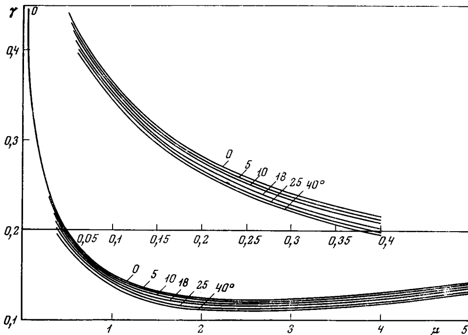
Рис. 14. Кривые изменения средних коэффициентов активности сульфата кальция в водных растворах в зависимости от ионной силы и температуры в интервале от 0 до 40° С
