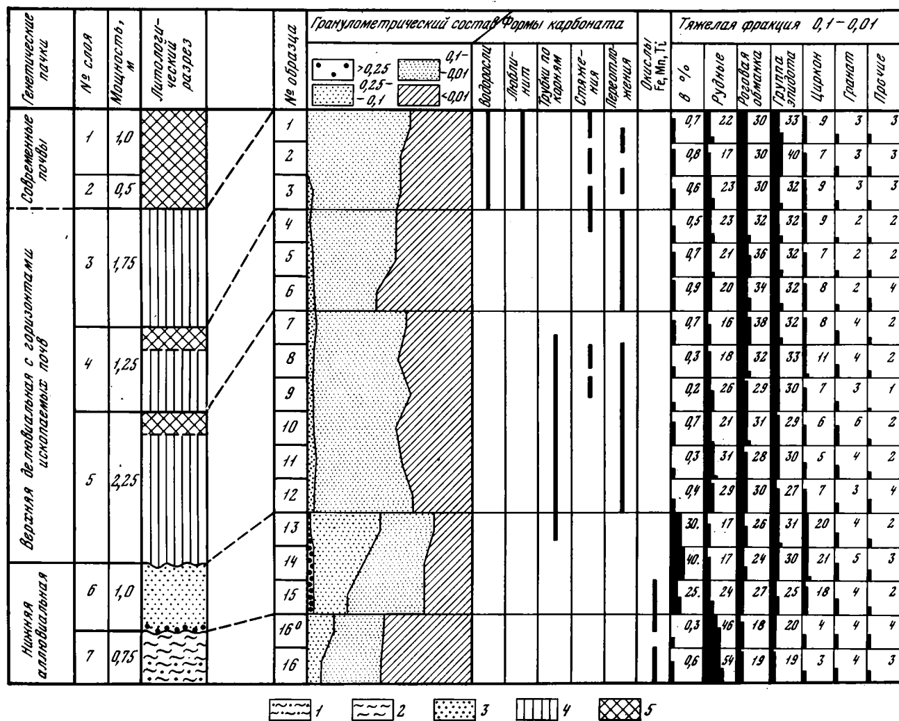
Рис. 1. Литолого-минералогическая характеристика отложений II террасы р. Лаба близ станции Темиргоевская
