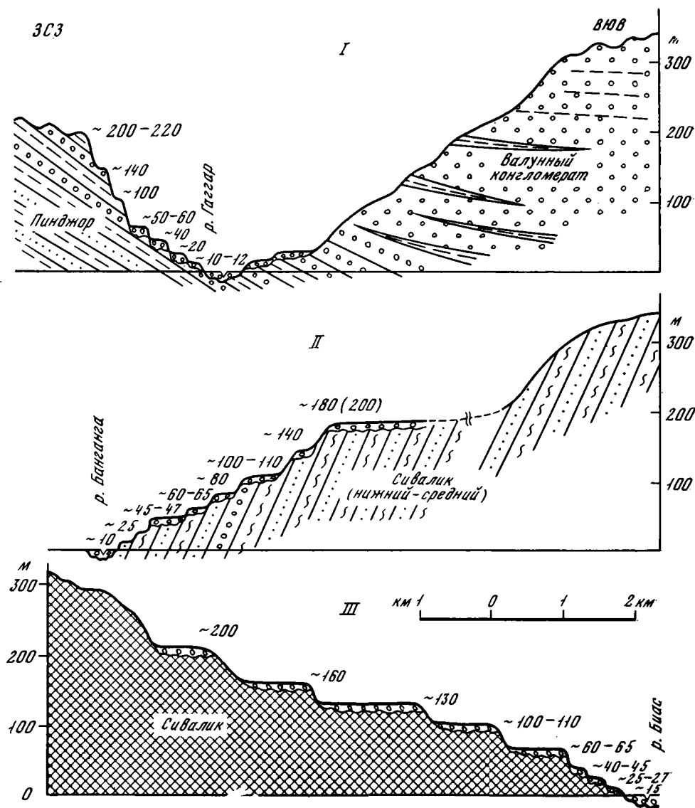
Рис. 4. Схематические геолого-геоморфологические профили долин рек
