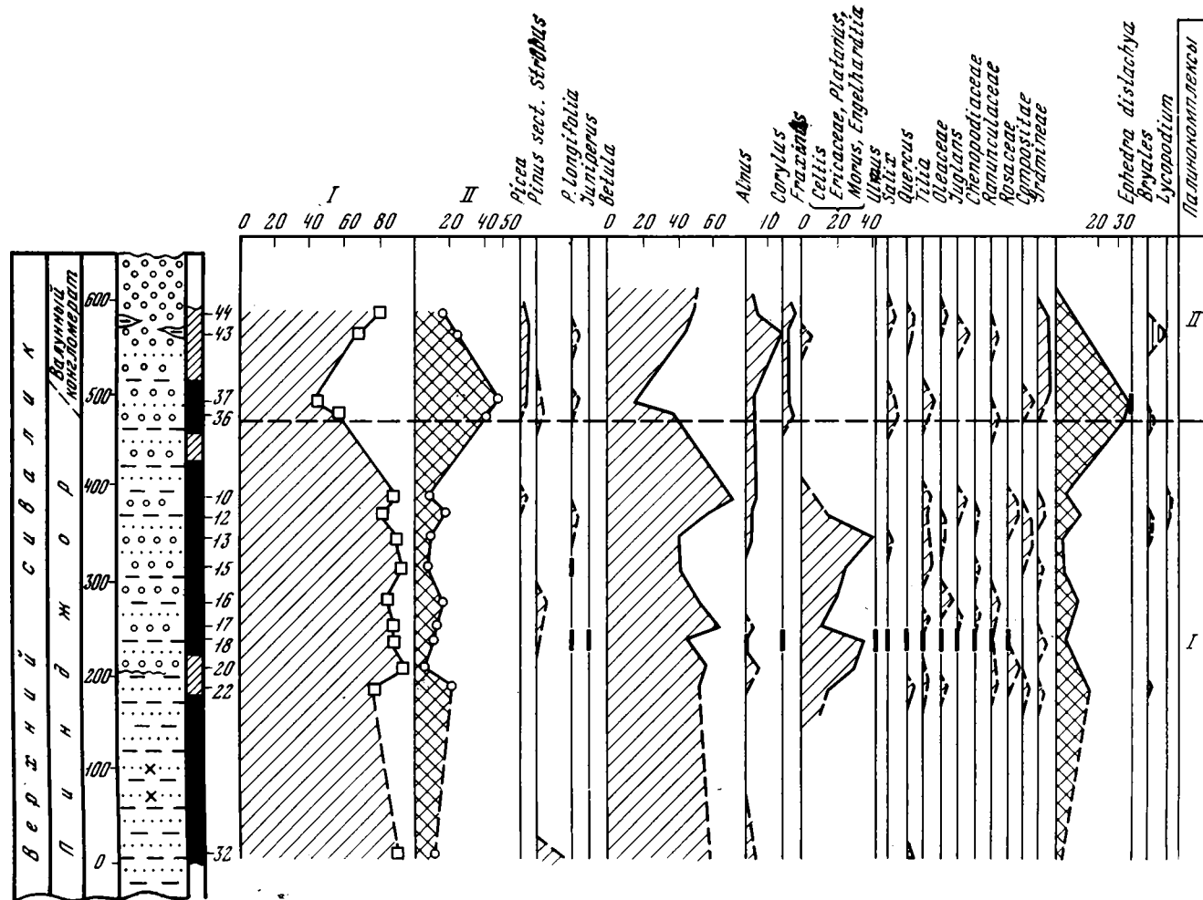
Рис. 3. Спорово-пыльцевая диаграмма верхнесиваликских отложений
