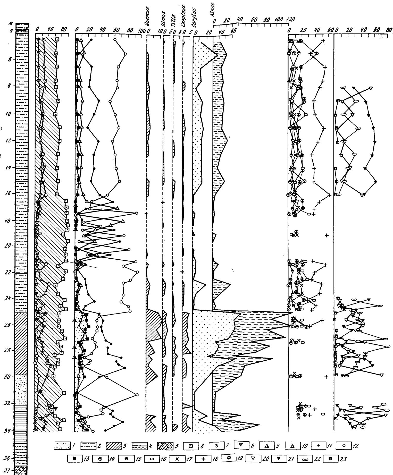
Рис. 2. Спорово-пыльцевая диаграмма древнеозерных отложений разреза у д. Горелово
