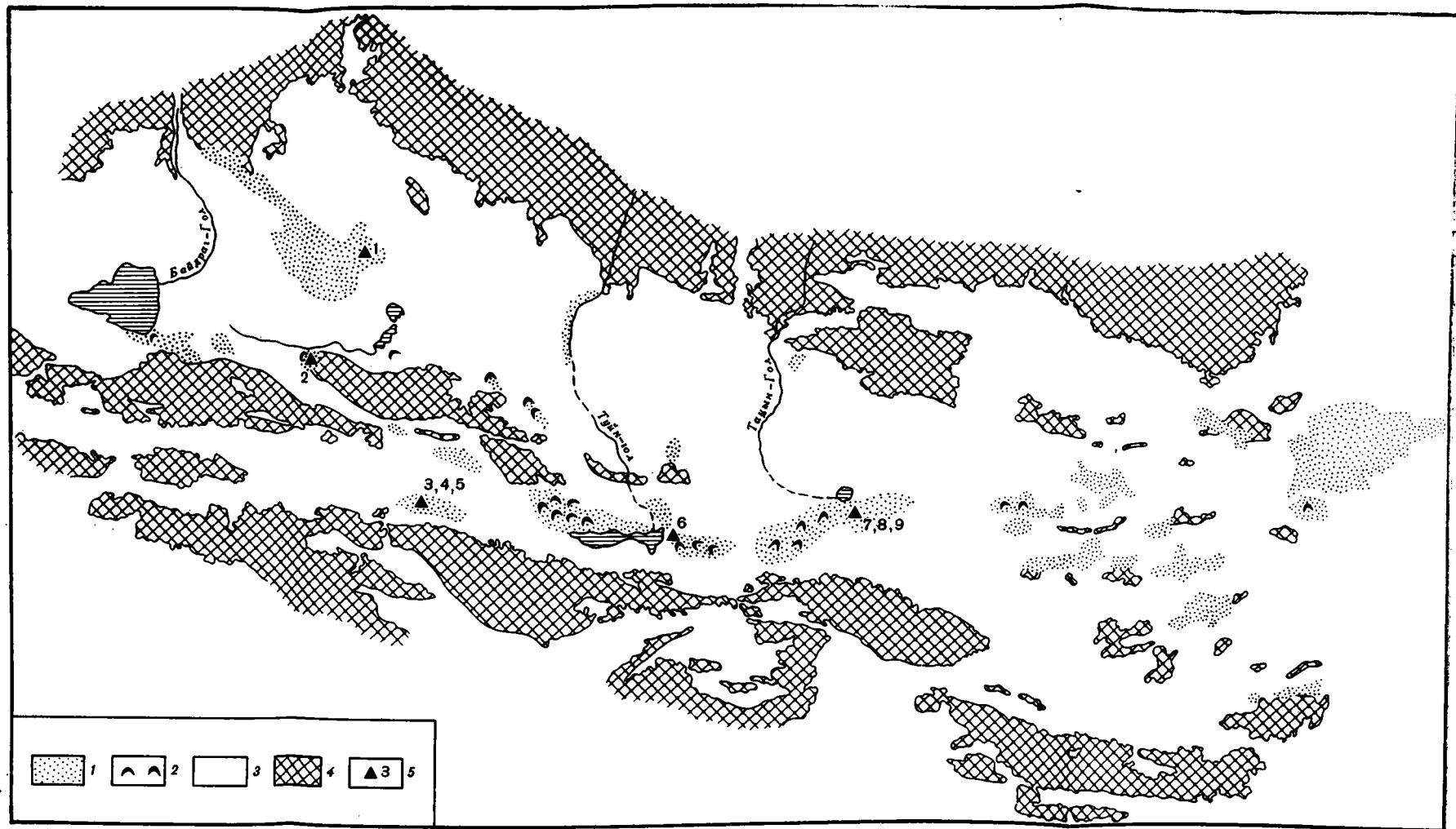
Схема распространения эоловых песков в Долине Озер (МНР)
