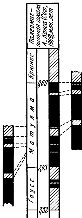
Рис. 5. Схема сопоставления палеомагнитной колонки отложений пинджора и нижней части валунных конгломератов с палеомагнитной шкалой А. Кокса [Сох, 1969]
