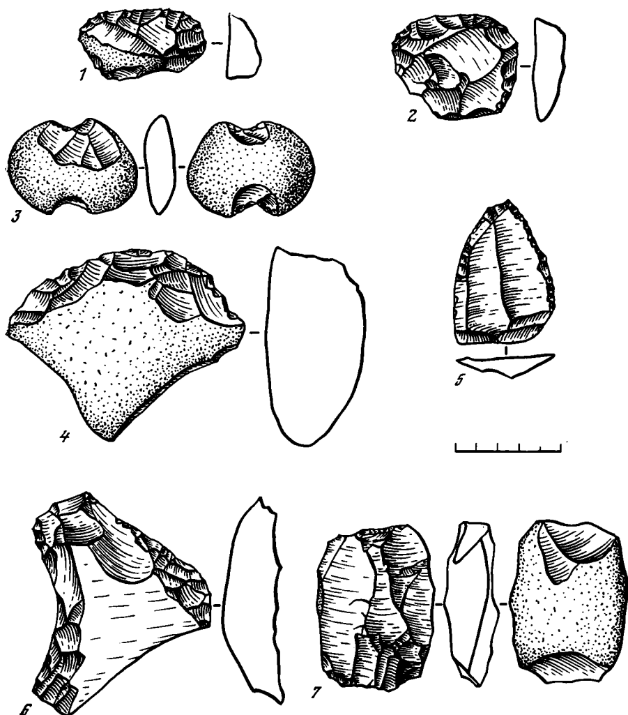
Рис. 1. Каменные изделия, собранные на высоких террасах Енисея
