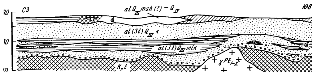
Рис. 2. Геологический разрез вдоль русла р. Гаврило
