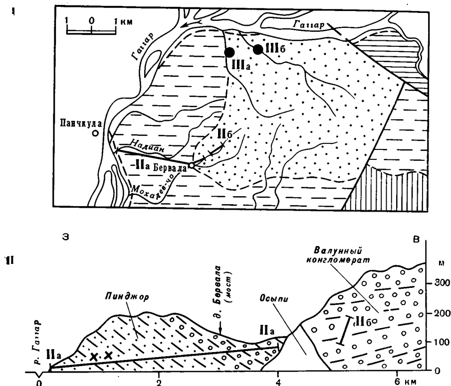
Рис. 2. Геологический разрез Могинанд (II) и его положение в бассейне р. Гаггар (I) Условные обозначения см. рис. 1. Геологическая карта дана по материалам Б. Тевари и А. Нанда [1968]
