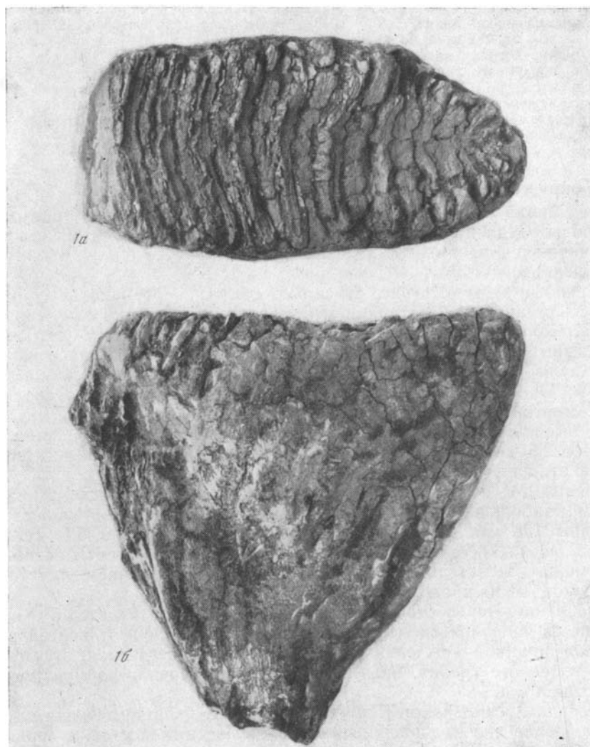
Рис. 4. Последние верхнечелюстные коренные зубы Mammuthus trogontherii chosaricus Dubrovo
