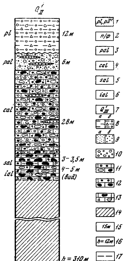
Рис. 1. Схематизированные разрезы отложений разновозрастных циклов террас р. Зеравшан
