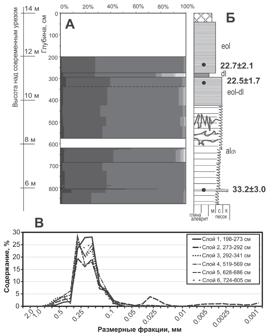
Рис. 9. Разрез Тк-1 (14–16-м «первая» терраса р. Хопер)
