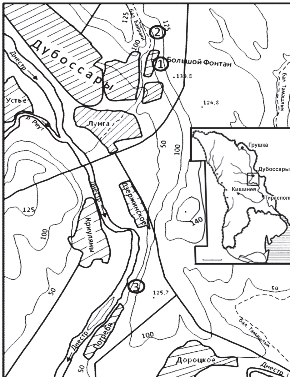
Рис. 1. Карта расположения ранне-палеолитических стоянок в районе г. Дубоссары 1 – Большой Фонтан; 2 – Байраки; 3 – Погребя
