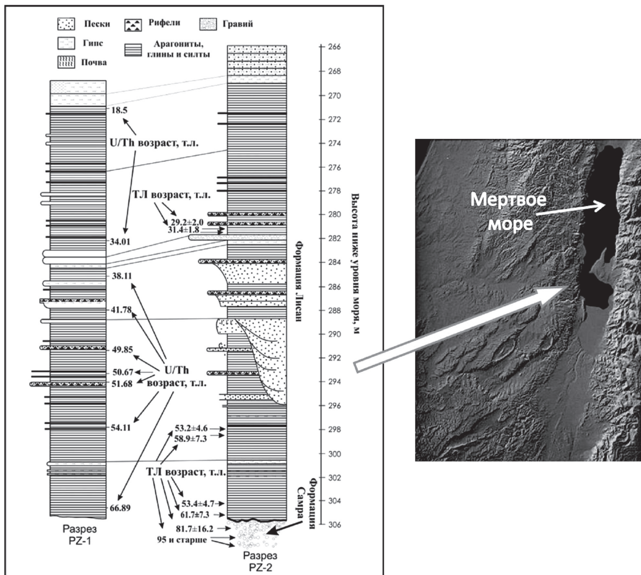
Рис. 19. Тестирование данных датирования регионально-эталонной технологии ТЛ анализа на классических разрезах Мертвого моря посредством их сравнения с результатами U/Th возрастных определений по [Stein, M. et al., 1997]
