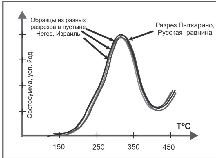
Рис. 17. ТЛ пики из насыщенных эталонов Русской равнины и пустыни Негев
