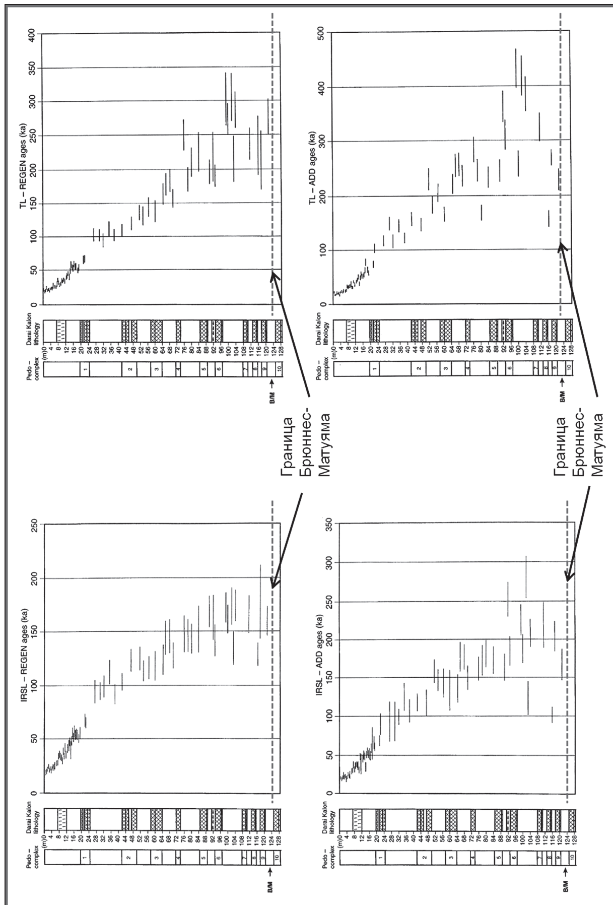
Рис. 15. Появление неправдоподобных датировок, получаемых посредством традиционной технологии ТЛ и ОСЛ датирования по [Friesen, Dodonov, 1998] – пояснения в тексте.
