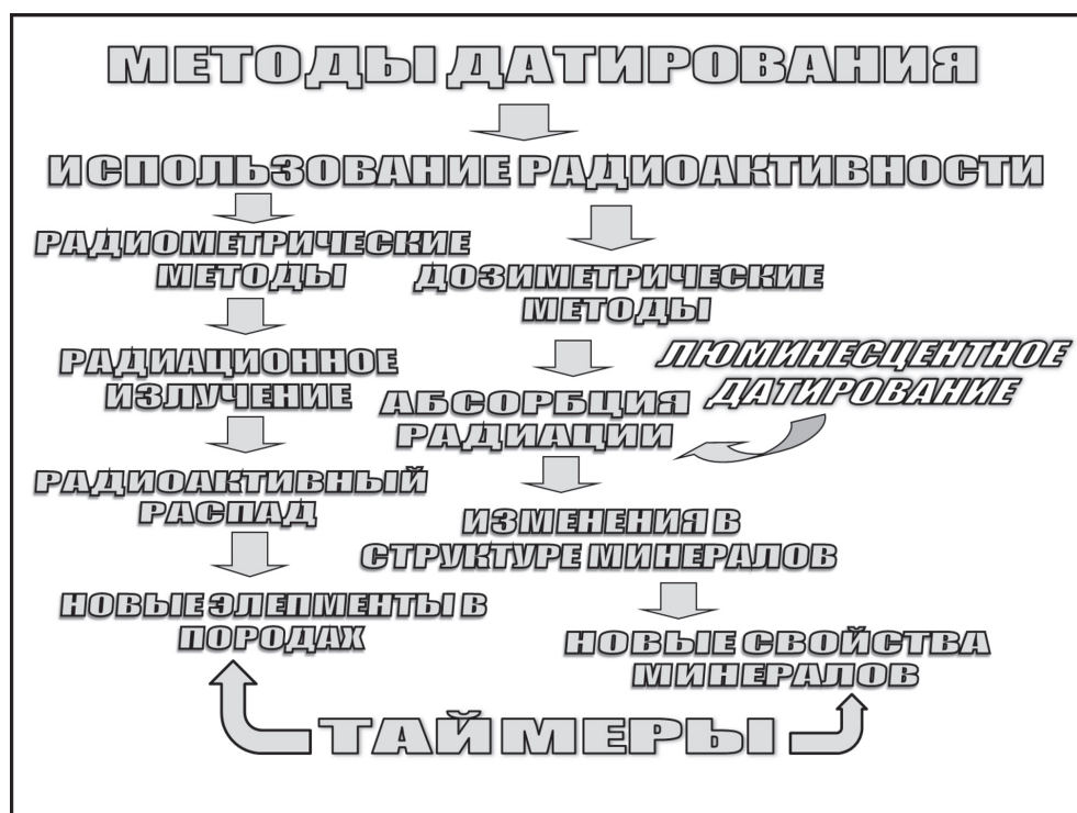
Рис. 1. Схема соподчиненности методов абсолютного датирования горных пород и используемых ими свойств радиоактивности
