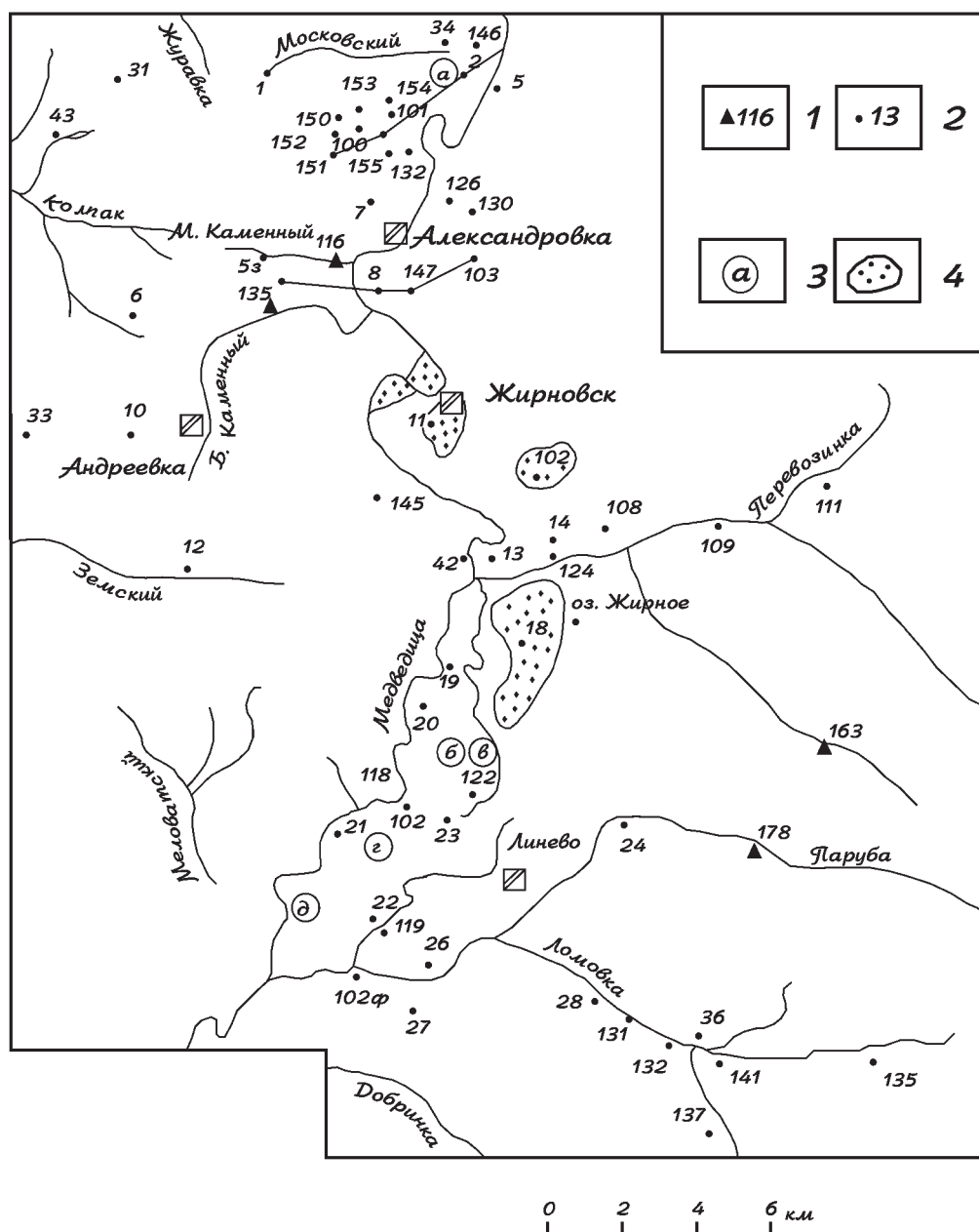
Рис. 1. Расположение обнажений и скважин на площади среднего течения р. Медведицы 1 – обнажения; 2 – скважины; 3 – озера: а – Подпесочное; б – Перекопское; в – Чеканное; г – Коньково; д – Глубокое; 4 – эоловые пески
