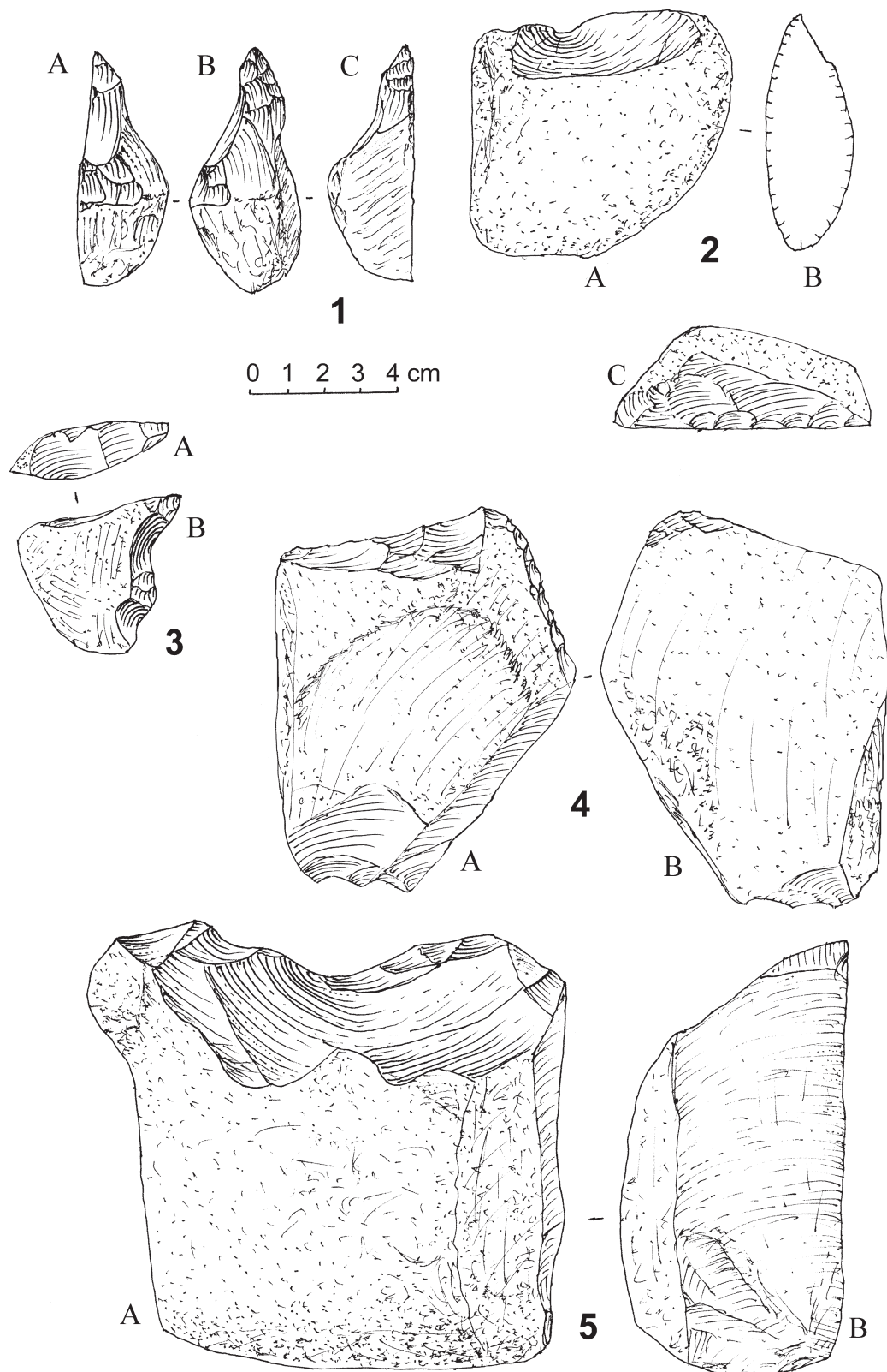
Рис. 5. Байраки. Каменные изделия аллювиального комплекса
