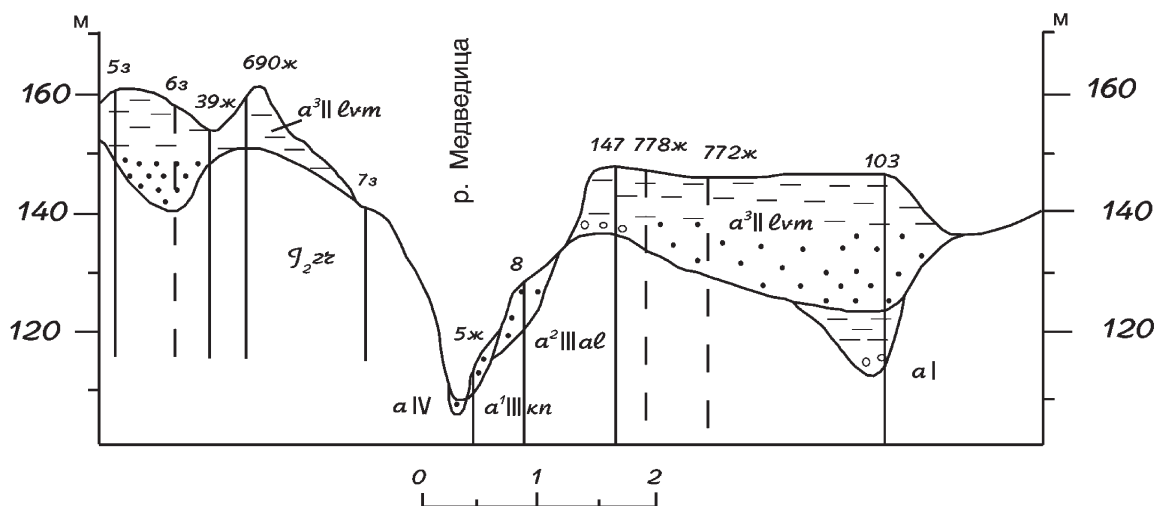
Рис. 3. Взаимоотношения разновозрастных аллювиальных отложений в долине Медведицы Условные обозначения – см. на рис. 2
