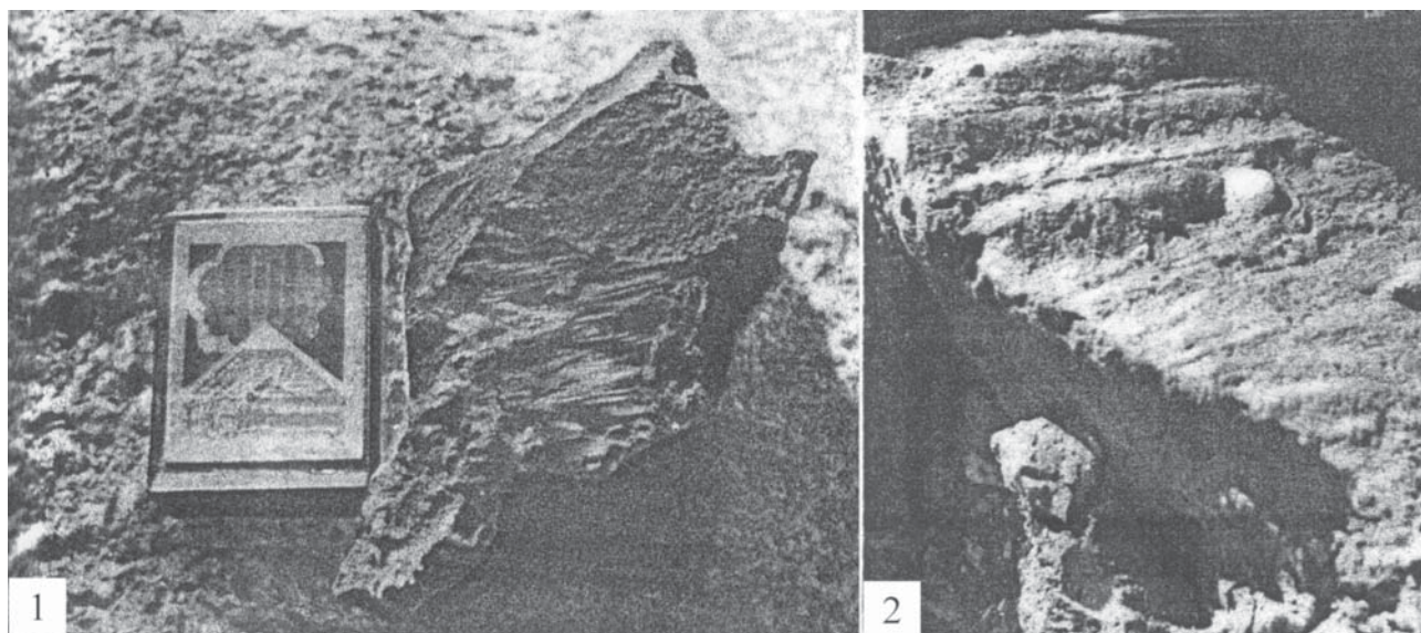
Рис. 7. Отражение процессов скольжения в виде линейных знаков скольжения разного масштаба в толщах плитчатых морен
