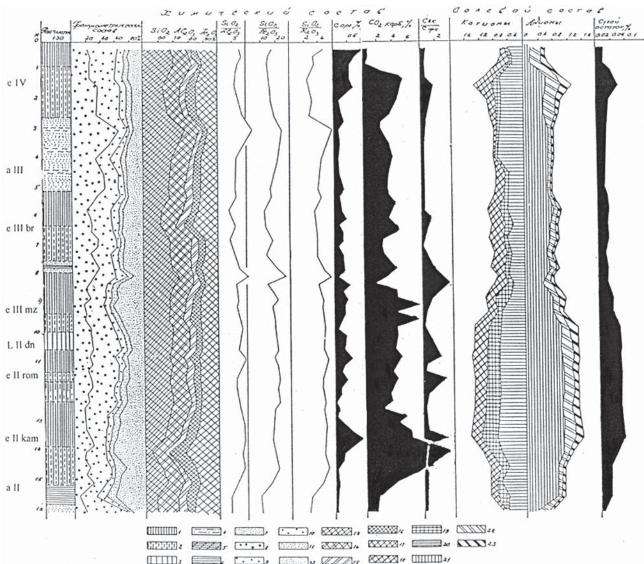
Рис. 9. Стратиграфическая колонка и вещественный состав плейстоценовых отложений разреза Рыбная Слобода
