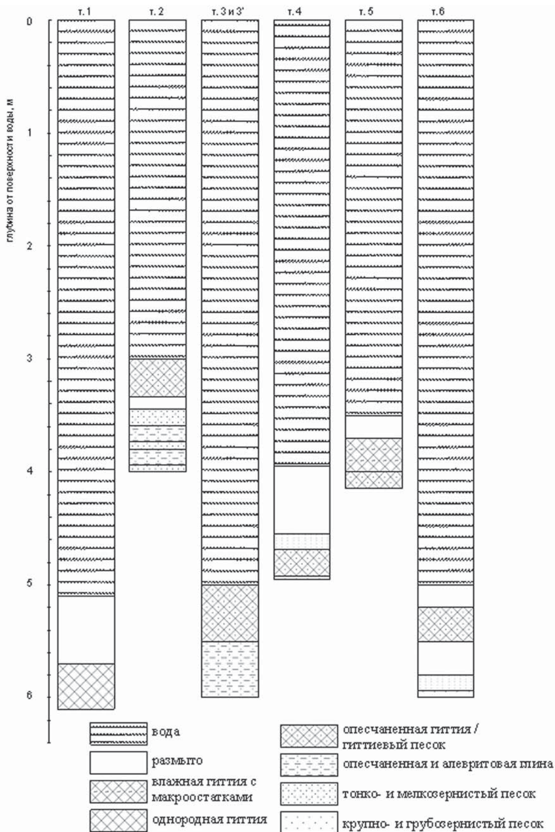
Рис. 13. Литостратиграфия донных отложений оз. Белого Fig. 13. Lithostratigraphy of lake sediments of the Lake Beloye
