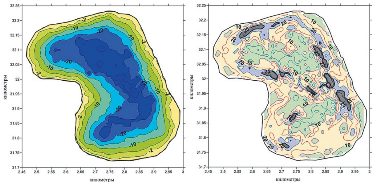
Рис. 3. Распределение глубин и уклонов дна оз. Белого.
