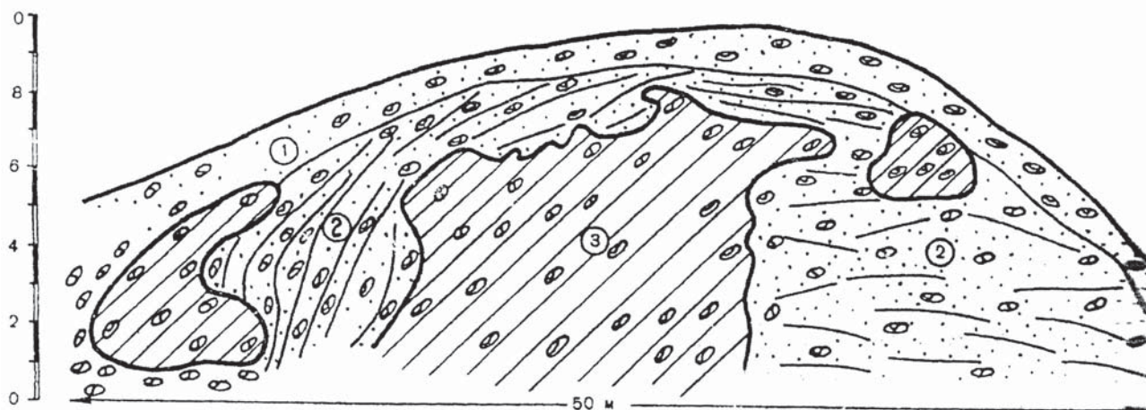
Рис. 4. Строение камового холма
