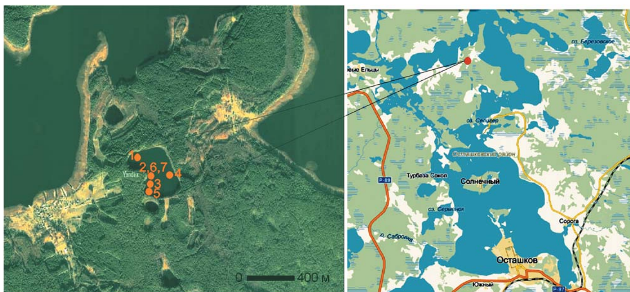
Рис. 2. Местоположение точек пробоотбора на оз. Белом Fig. 2. Location of the sampling points on the Lake Belaye
