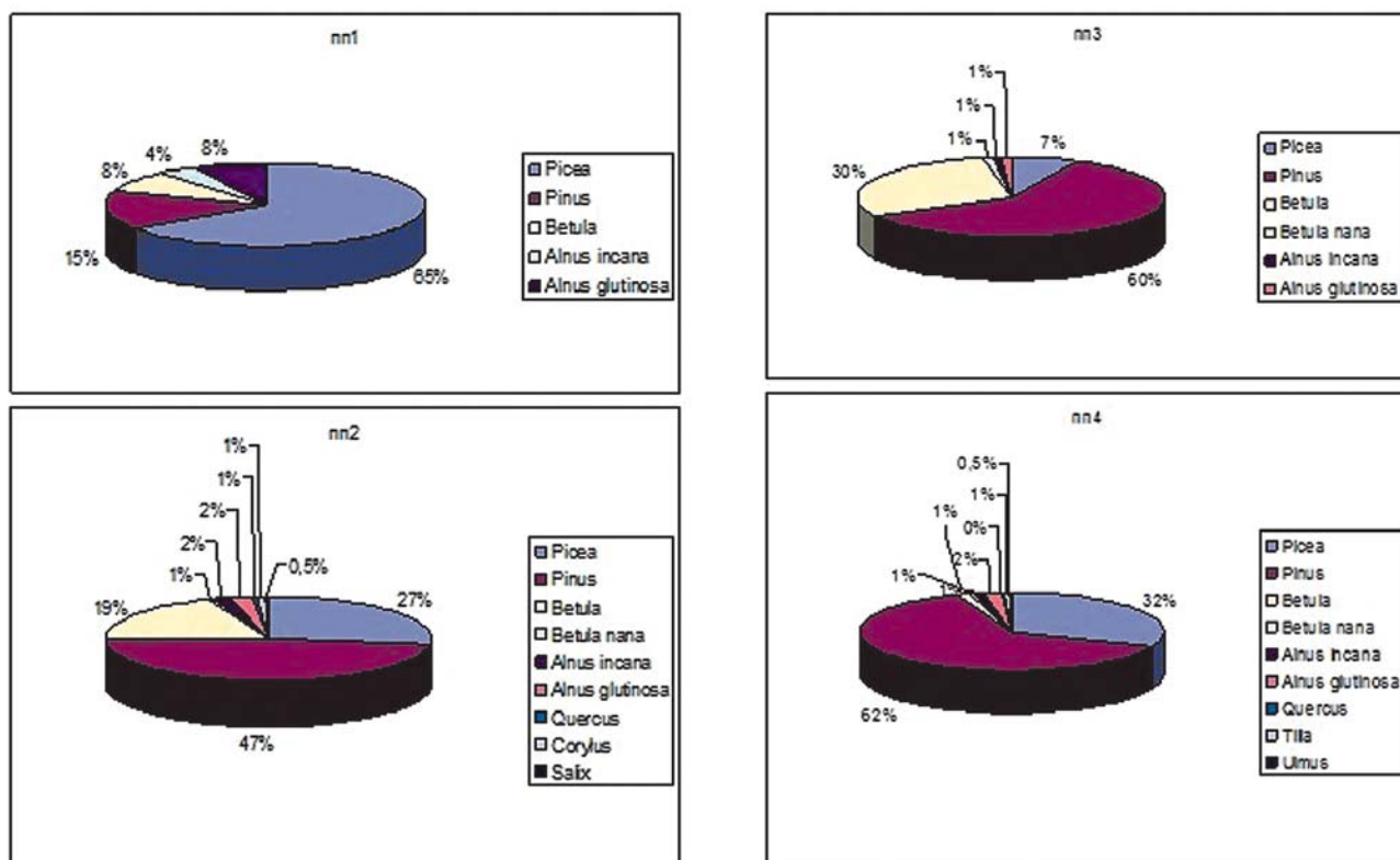
Рис. 10. Процентное содержание пыльцы древесных пород в поверхностных пробах озер Белого и Черного Fig. 10. Percentage of tree pollen in surface samples from lakes Beloye and Chernoye
