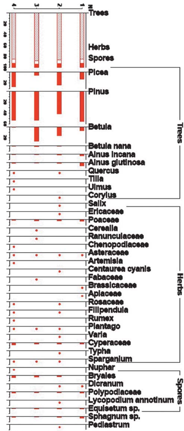
Рис. 9. Спорово-пыльцевая диаграмма поверхностных проб озер Белого и Черного. Слева указаны номера проб.
