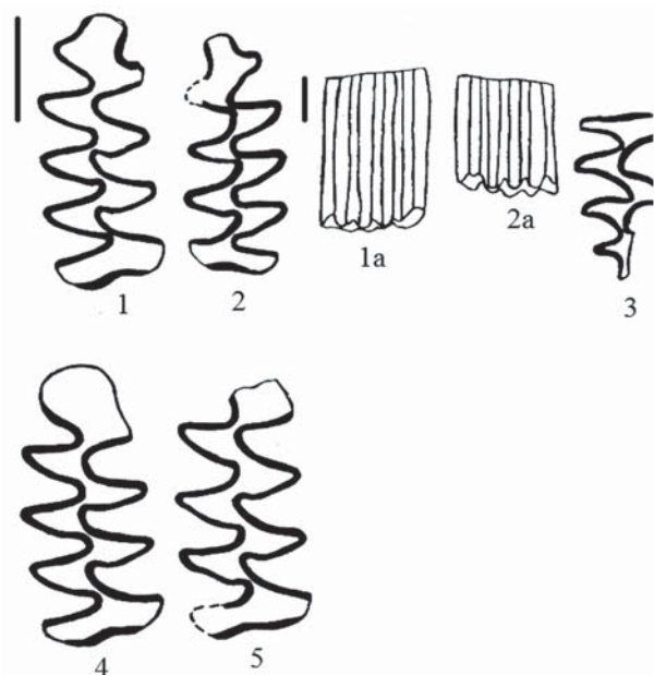
Рис. 6. 1, 2 – м1, 3 – М3 степной пеструшки Lagurus transiens ; 4, 5 – м1 желтой пеструшки Eolagurus luteus volgensis
