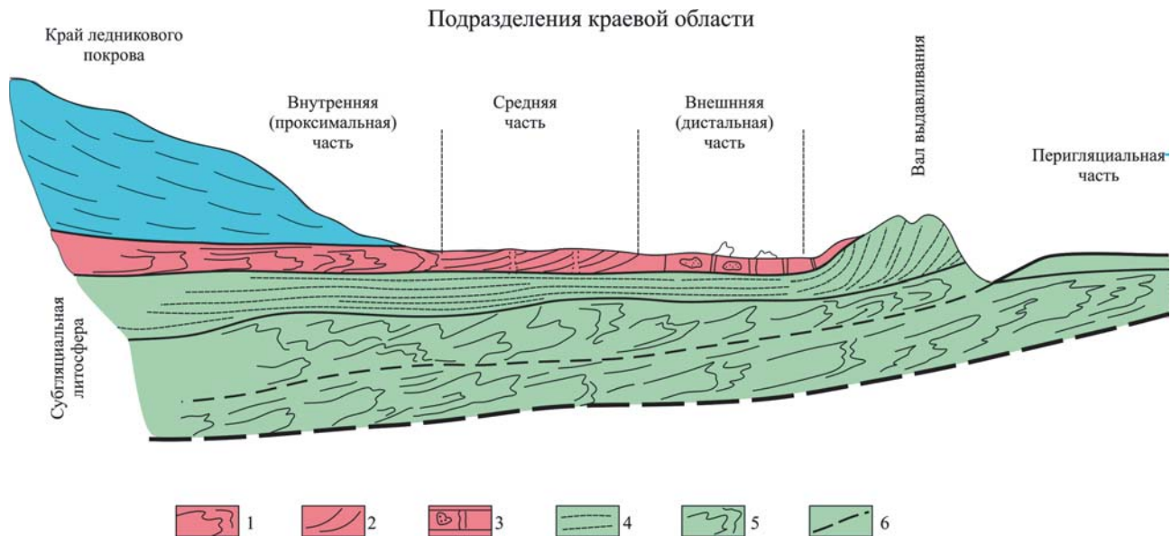
Рис. 1. Принципиальная схема строения краевой зоны покровного оледенения
