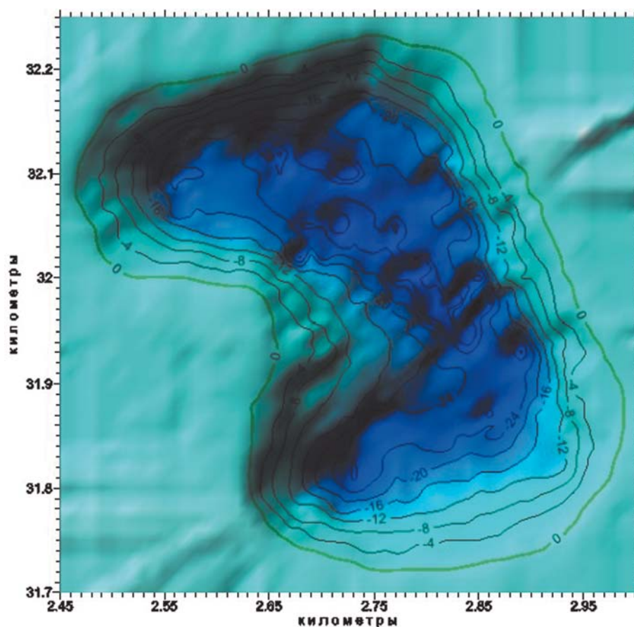
Рис. 8. Трехмерная модель оз. Белого Fig. 8. Three-dimensional model of the Lake Belaye
