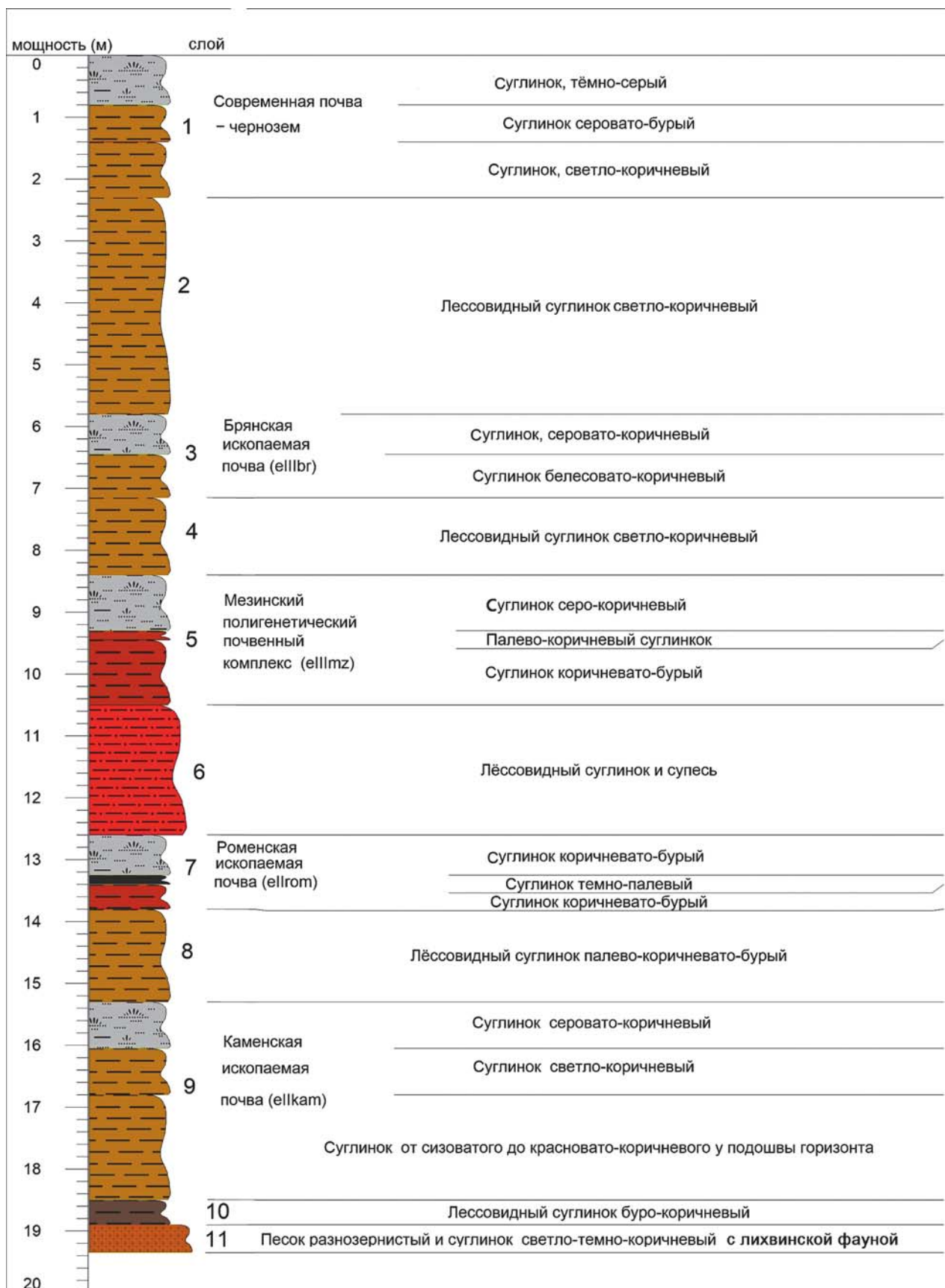
Рис. 2. Структура и состав отложений разреза Рыбная Слобода.
