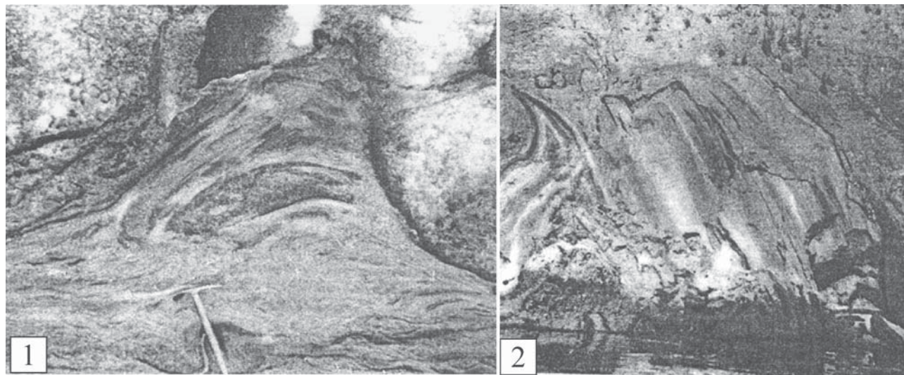
Рис. 2. Гляциодиапиры в толще мореносодержащего льда в Гренландии (1) и в строении морены М-2 в районе г. Углича (2).
