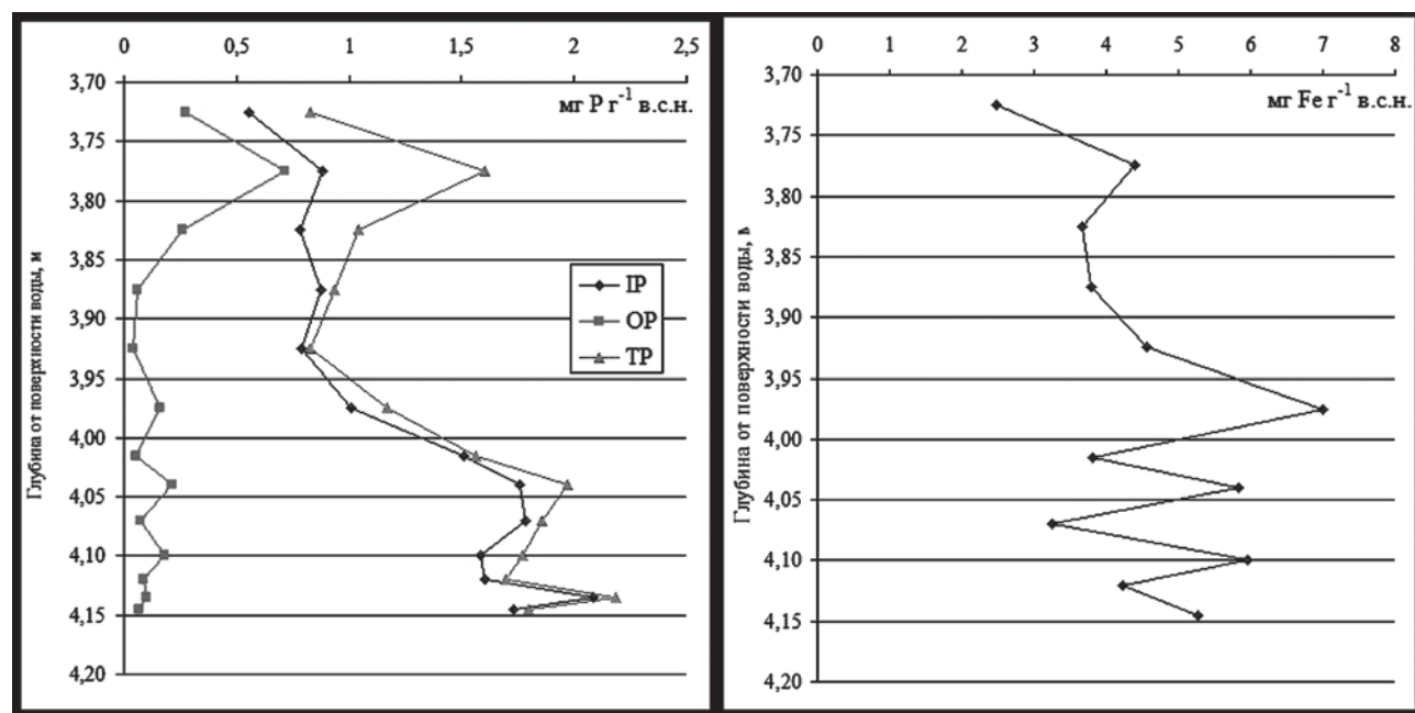
Рис. 17. Вертикальное распределение фосфора (а) и железа (б) в колонке донных отложений оз. Белого Fig. 17. Vertical distribution of phosphorus (a) and Fe (b) in the lake sediments of the Lake Beloye
