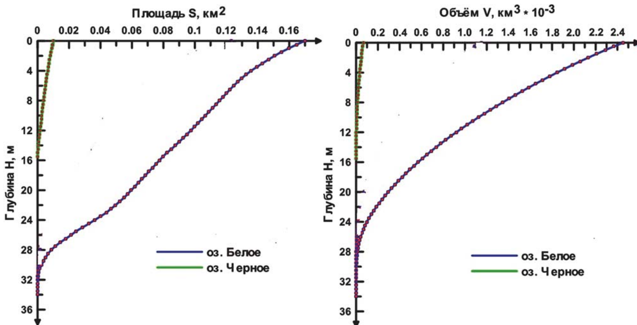
Рис. 5. Батиграфические и объемные кривые озер
