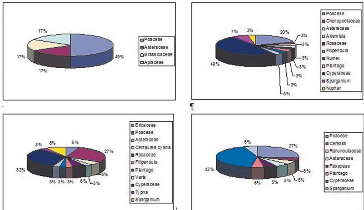
Рис. 11. Процентное содержание пыльцы трав в поверхностных пробах озер Белого и Черного Fig. 11. Percentage of herbs pollen in surface samples from lakes Beloye and Chernoye
