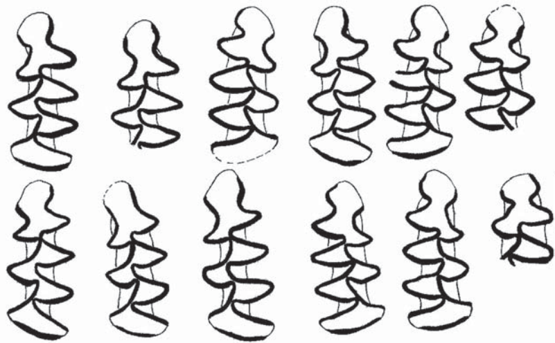
Рис. 3. Передние нижние моляры m1 водяной полевки Arvicola cantianus Fig. 3. First lower molars m1 of water vole Arvicola cantianus
