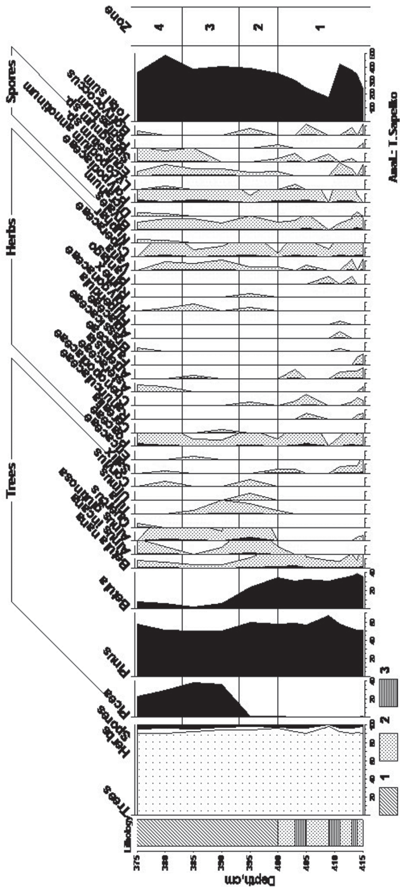
Рис. 15. Спорно-пыльцевая диаграмма оз. Белого. Условные обозначения: 1 — бурая гиття; 2 — песок; 3 — черная гиття
