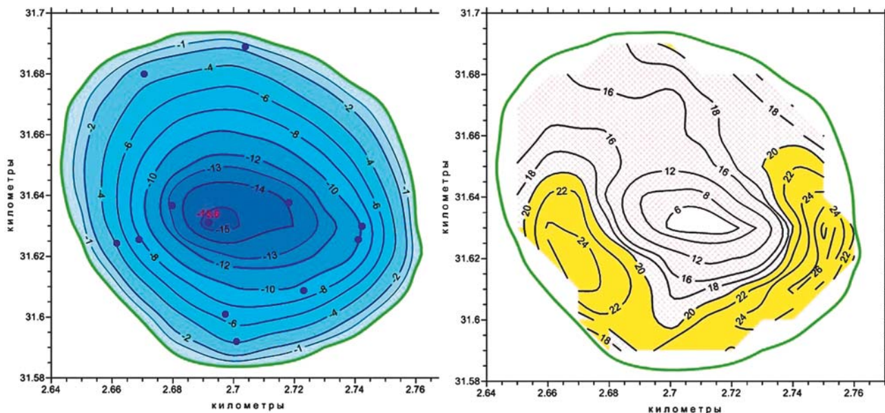
Рис. 4. Распределение глубин и уклонов дна озера Черного.
