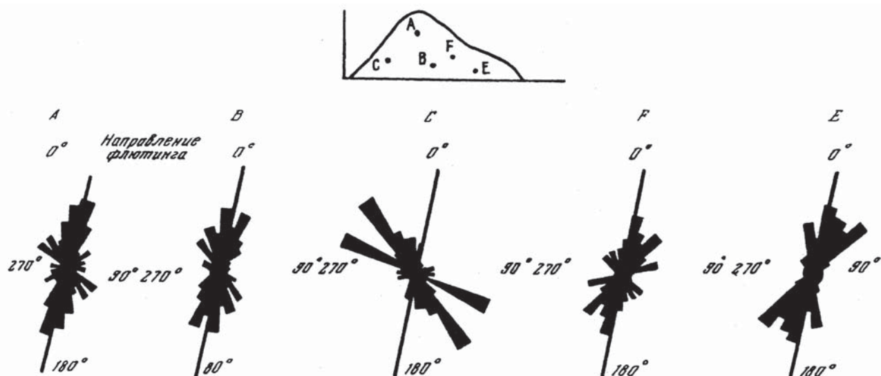
Рис. 8. Результаты исследования ориентировки удлиненных минеральных и гравийных частиц в одной из гряд – флютинга (по [Freschauf, 1971]).
