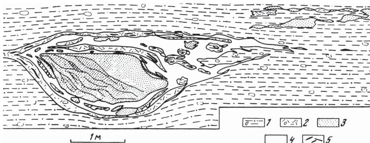
Рис. 5. Отторженец в толще морены М-2; в строении отторженца принимают участие четвертичные и меловые отложения – К-2, (пос. Алтыново, окрестности г. Углича).
