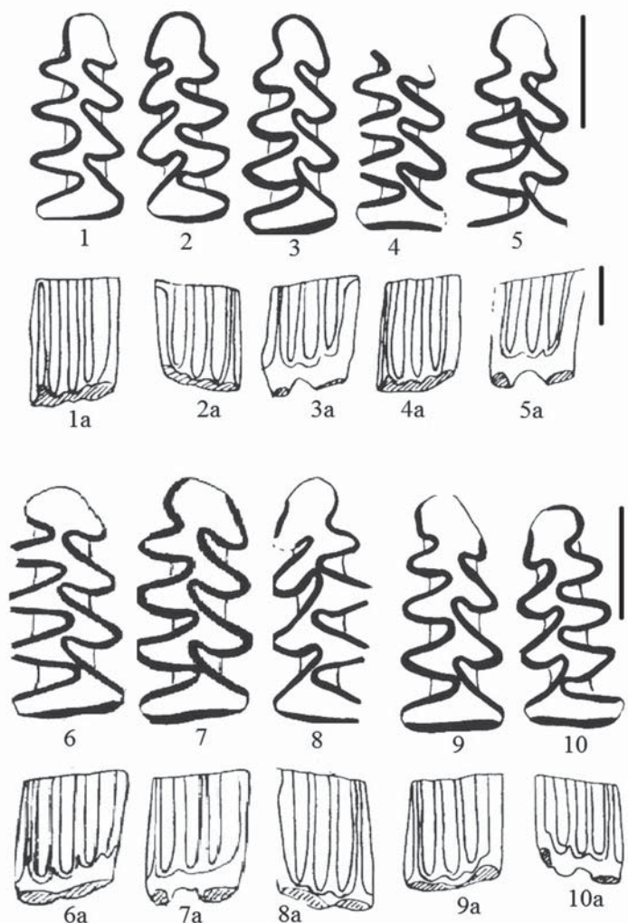
Рис. 8. 1–5 – жевательная поверхность m1, 1a–5a – боковая поверхность m1 Clethrionomys glareolus ; 6–10 – жевательная поверхность, 6a–10a – боковая поверхность m1 Clethrionomys rufocanus
