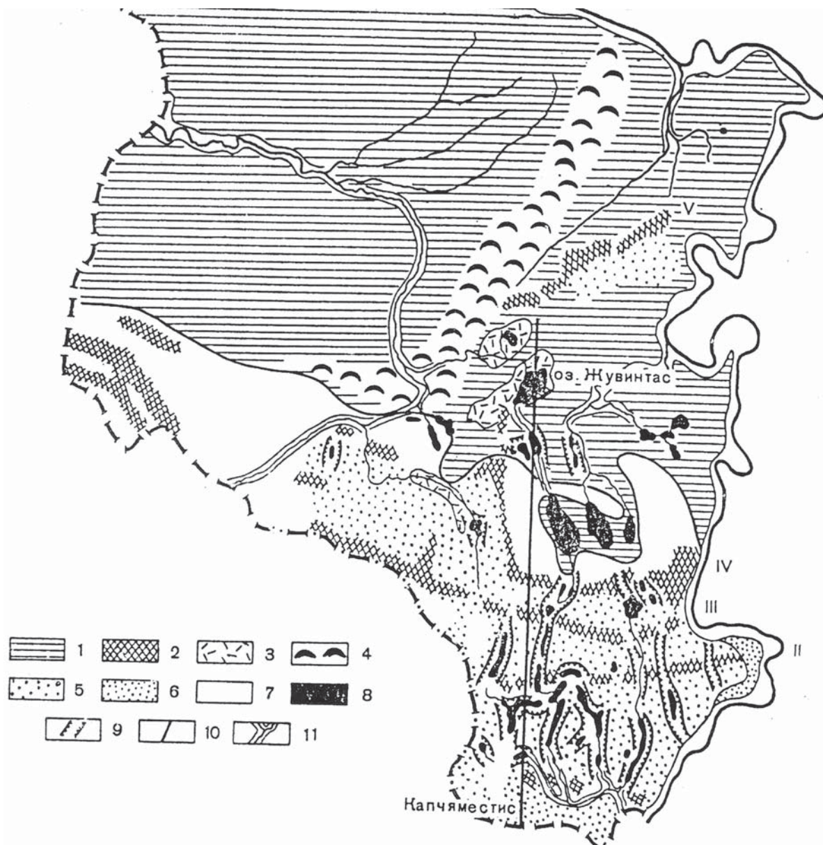
Рис. 3. Геоморфологическая схема Южной Литвы [Гарункштис, 1965]
