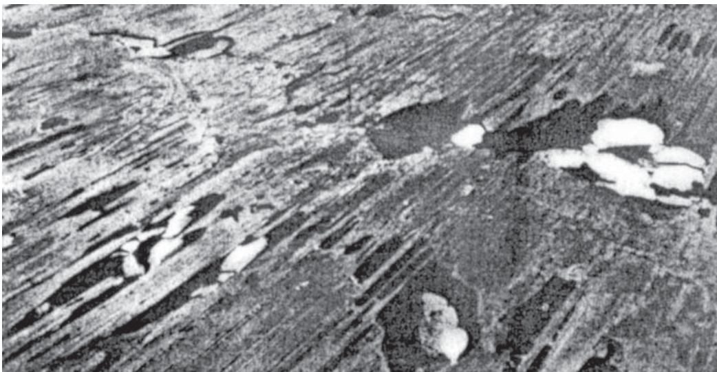
Рис. 6. Рельеф флютинг-морены, общий вид (Канада). Fig. 6. General view of fluting-till relief (Canada).
