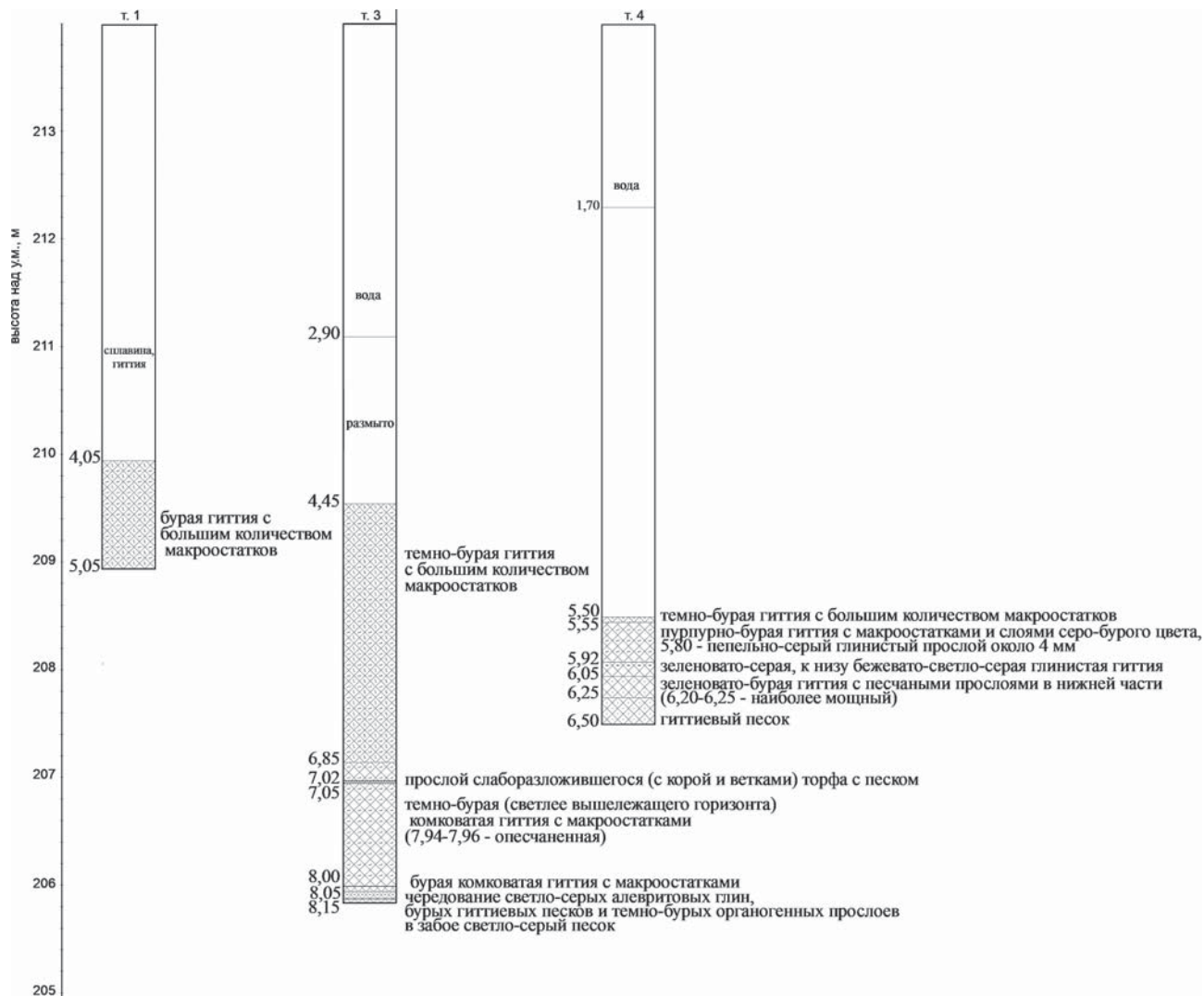
Рис. 14. Лито­стра­ти­гра­фия дон­ных от­ло­же­ний оз. Чер­но­го Fig. 14. Lithostratigraphy of lake sediments of the Lake Chernoye
