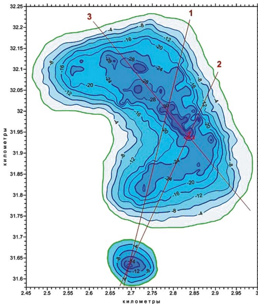
Рис. 6. Месторасположение разрезов на карте распределения глубин озёр Белое и Черное Fig. 6. The location of the sections on the map of the depth distribution of the lakes Beloye and Chernoye
