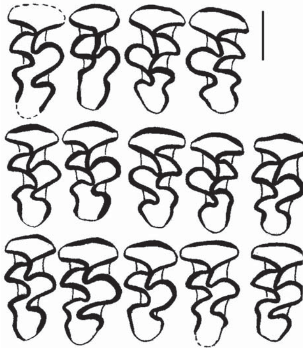
Рис. 4. Третьи верхние моляры M3 водяной полевки Arvicola cantianus Fig. 4. Third upper molars M3 of water vole Arvicola cantianus
