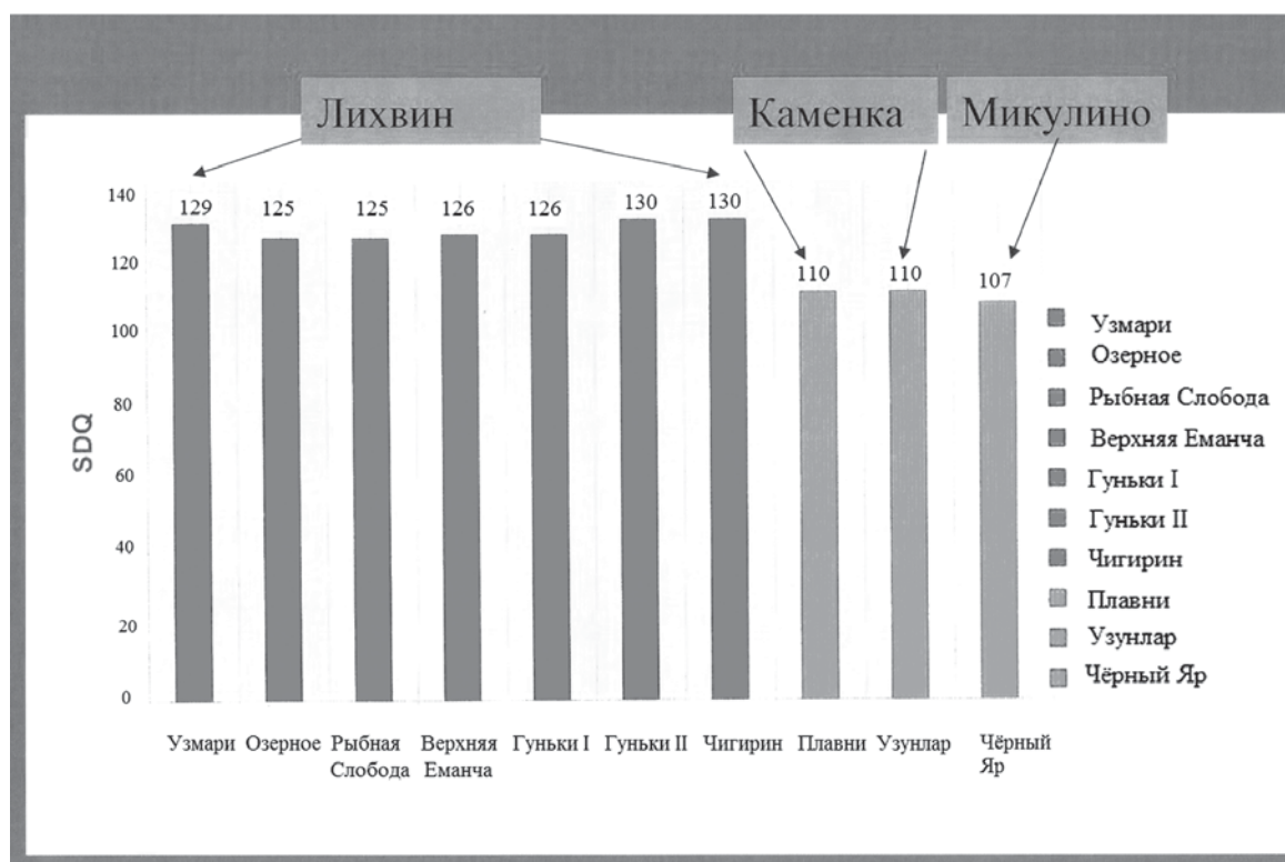
Рис. 5. SDQ индекс моляров Arvicola из отложений лихвинского, каменского и микулинского межледниковий Русской равнины
