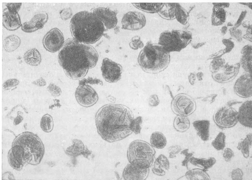
Рис. 8. Общий вид спорового состава отложений регрессий. 1 — петликовские споры; тинкий спора; вертикальный разрез. \times 150 ; 2 — нижнешироковские споры, \times 150 .
