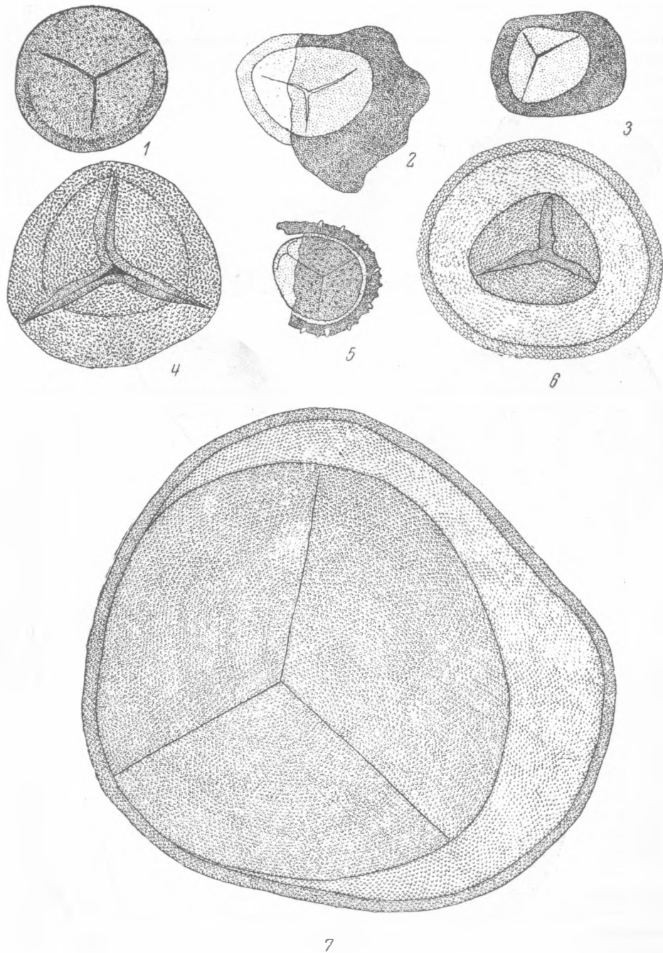
Рис. 3. Споры с плотным периспорием подгруппы Archaeozonotriletes Naum.
