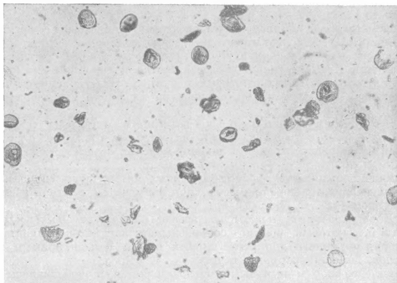
Рис. 7. Общий вид спорового состава отложений трансгрессий. 1 — рудкинские слои, \times 150 ; 2 — псковские слои, \times 150 .
