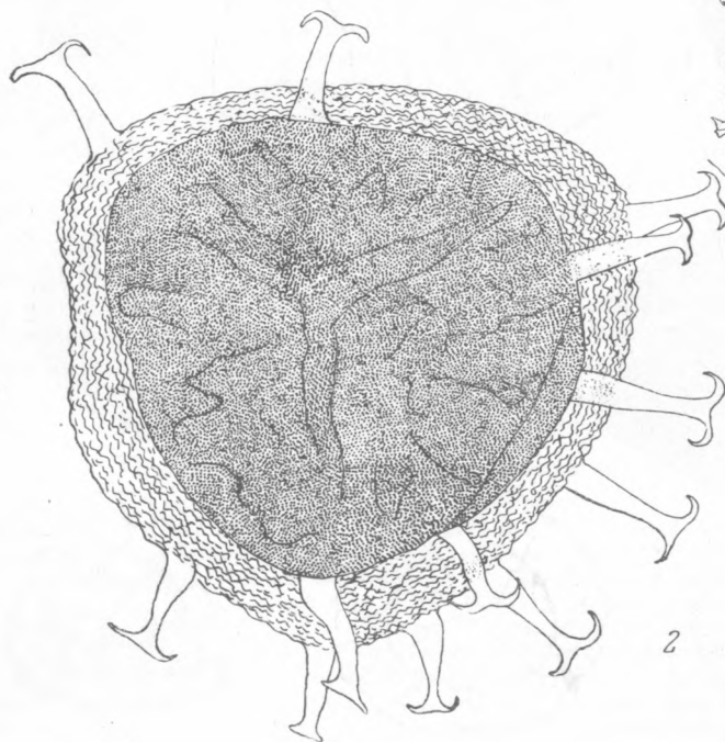
Рис. 2. Споры современные и ископаемые.
