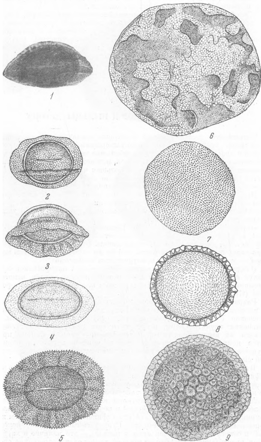
Рис. 5. Пыльца голосеменных верхнего девона.
