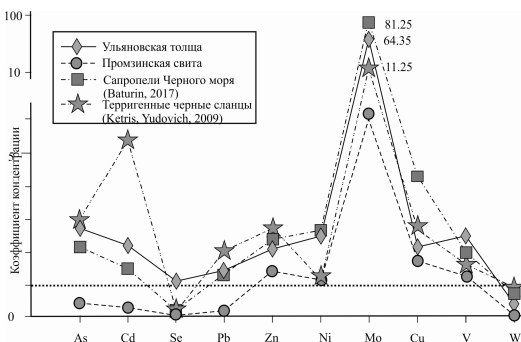
Рисунок. Коэффициенты концентрации токсичных элементов в нижеаптских, средневолжских и современных толщах, накопившихся в аноксических условиях в сопоставлении со средними содержаниями в глинах (Grigor'ev, 2003)
